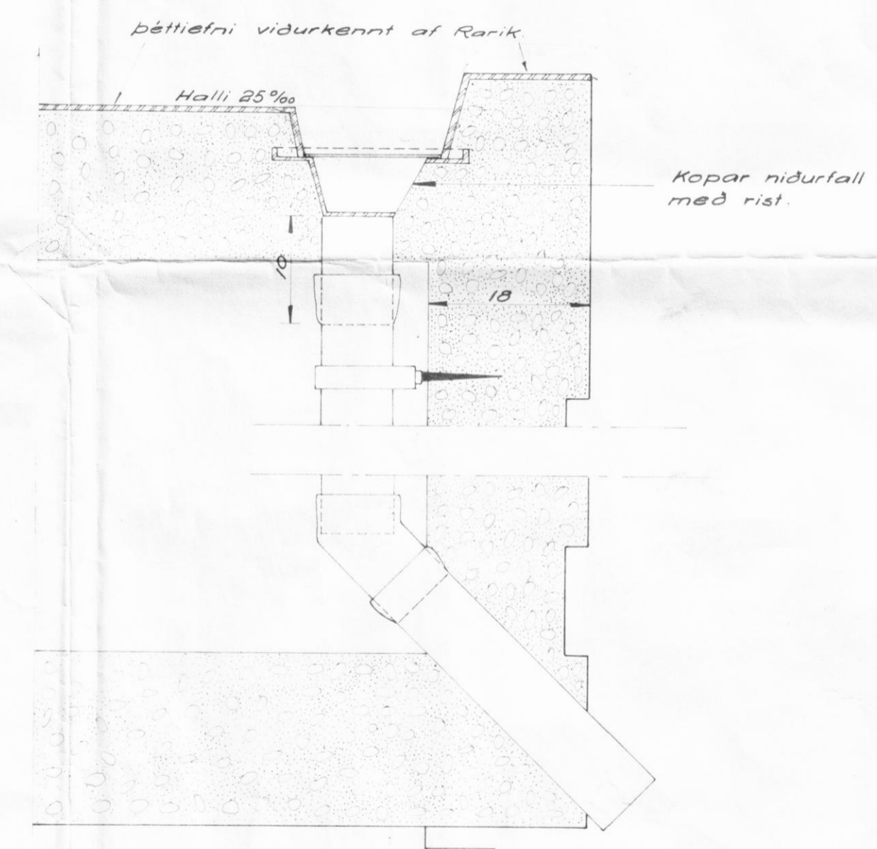
Frágangur á níðurfallsróri. M:1:5.
