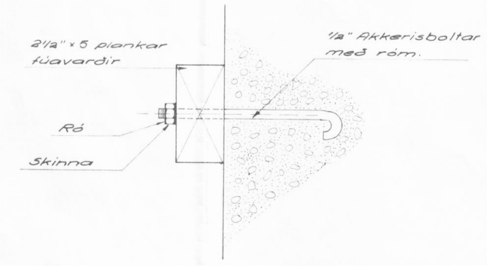
Festingar á plönkum. M:1:5.
