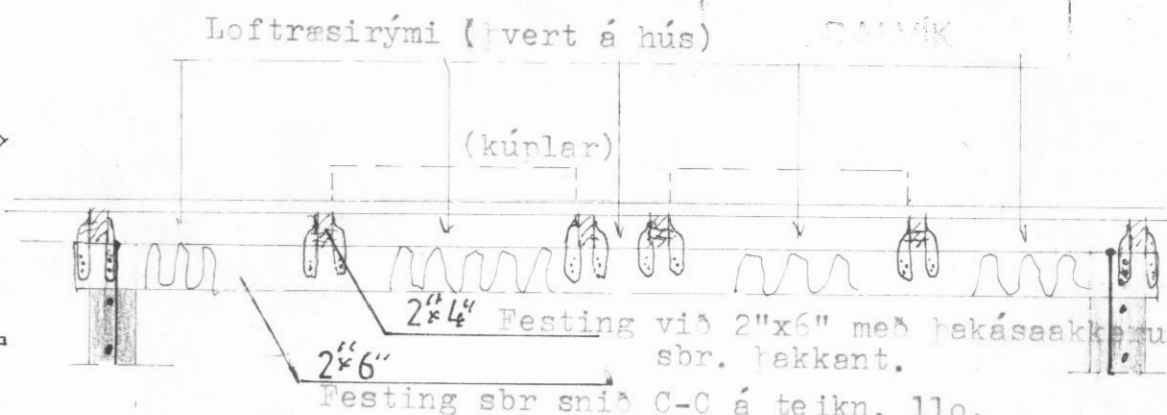
SNÍÐ T-T M. 1:25
