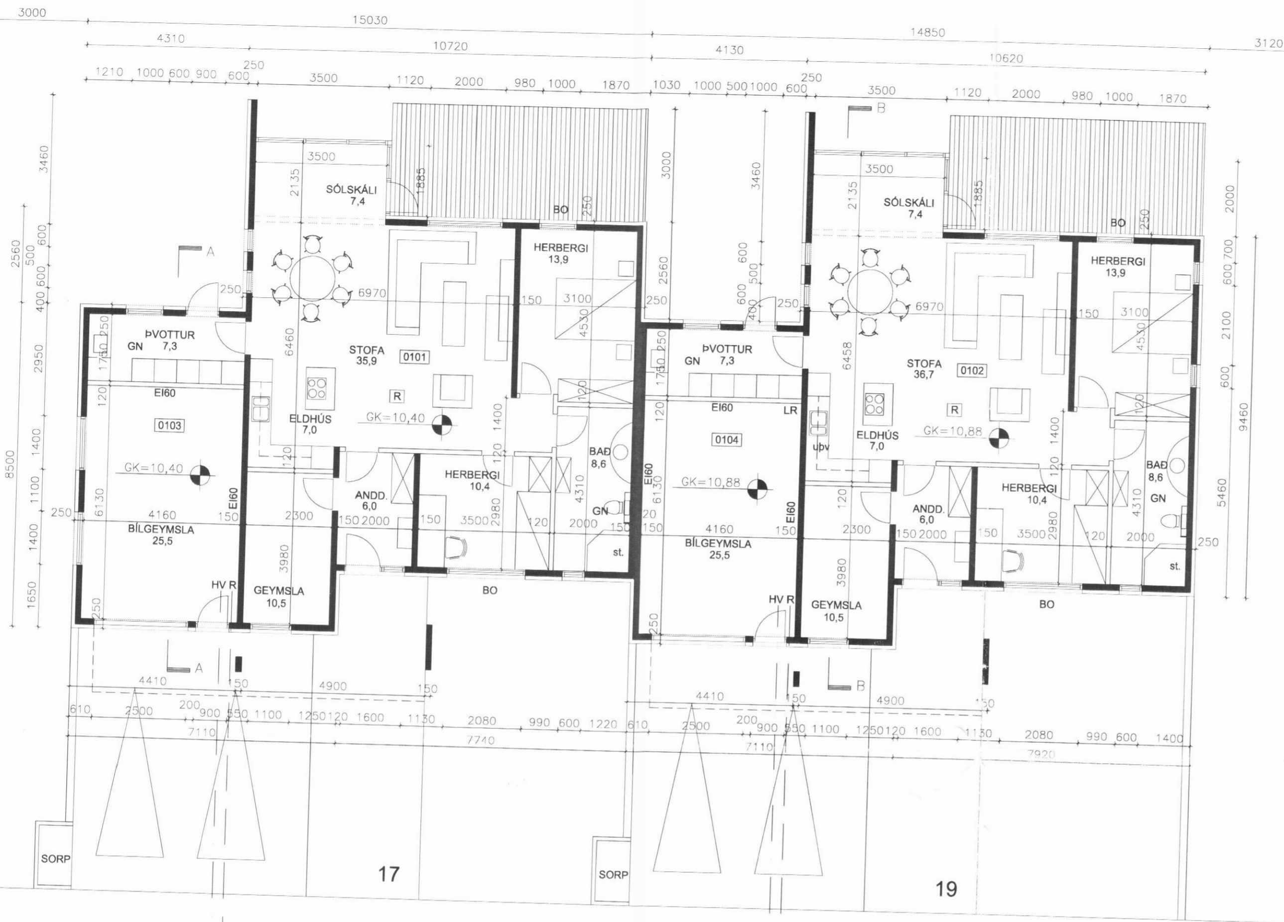
GRUNNMYND MKV. 1:100
