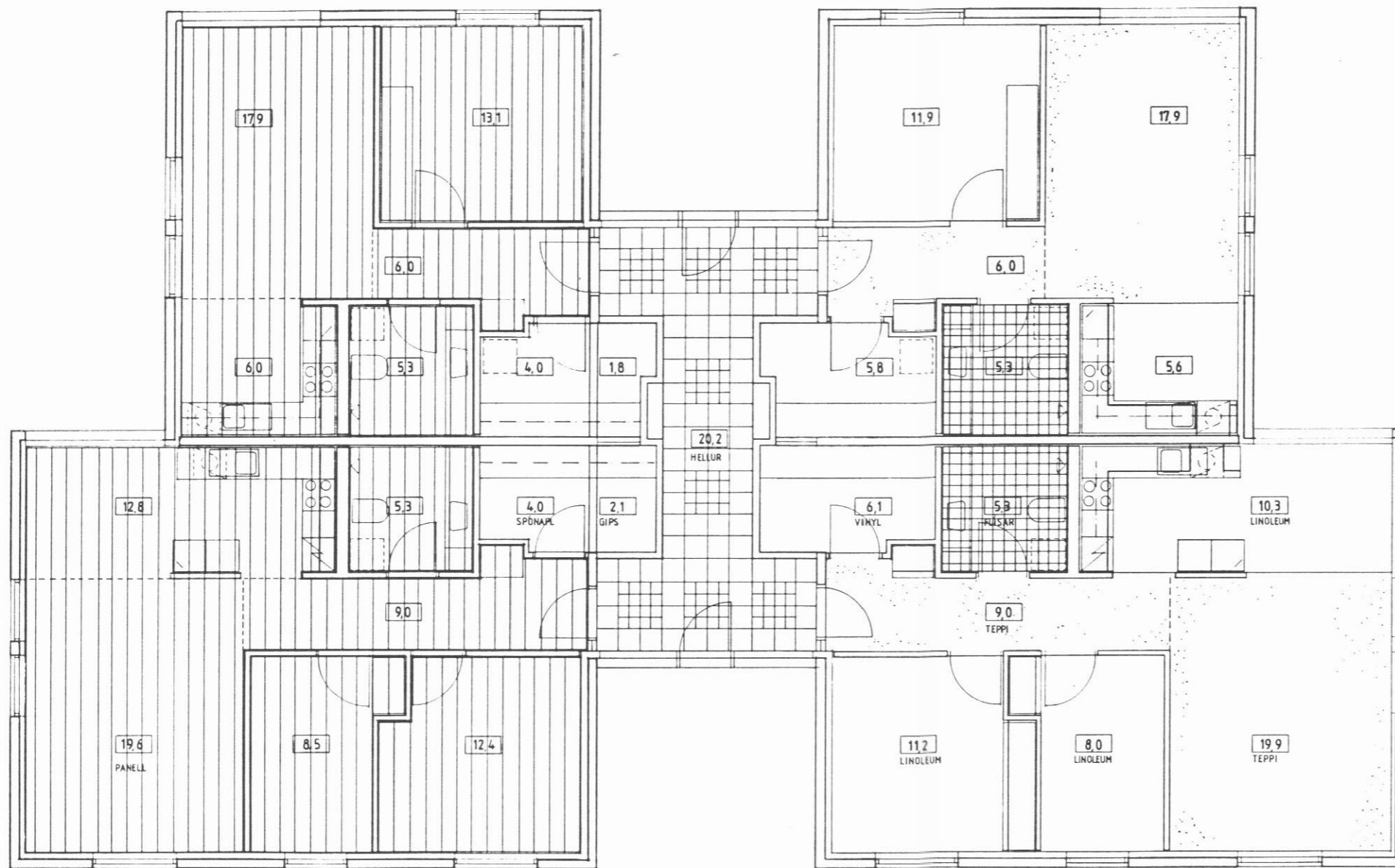
LOFTAEFNI Grunnmynd
