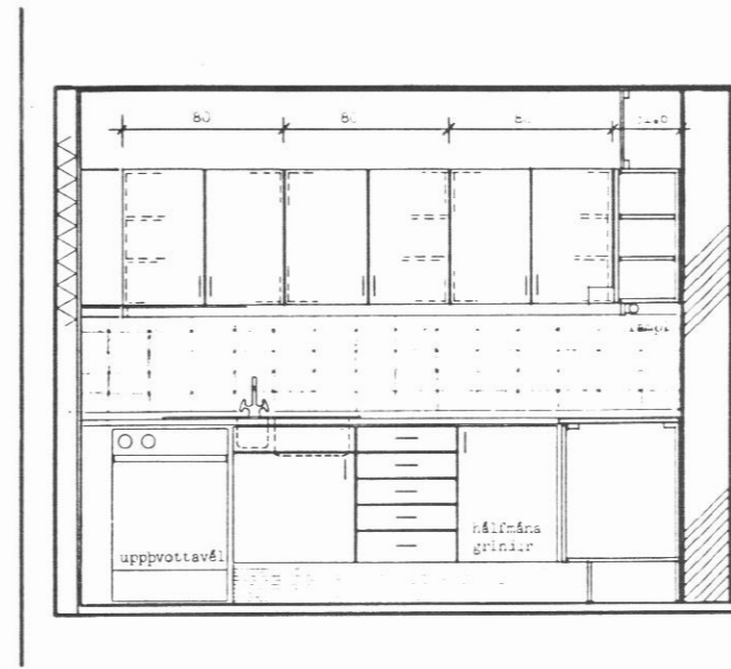
SNID A-A
