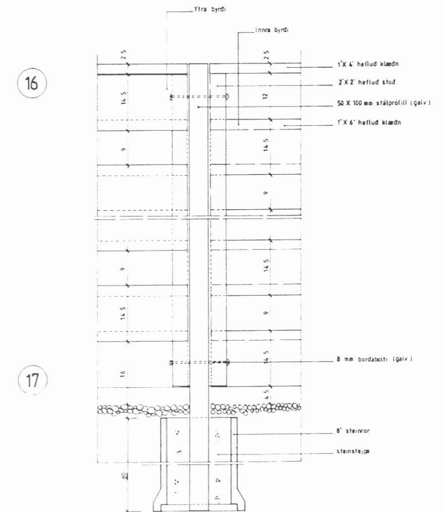
Lódrétt deili í skjólvegg m. 1:5
