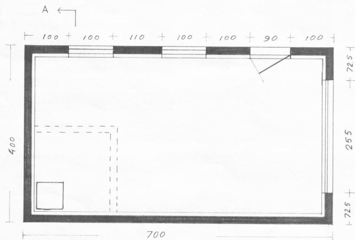
Grunnmynd
