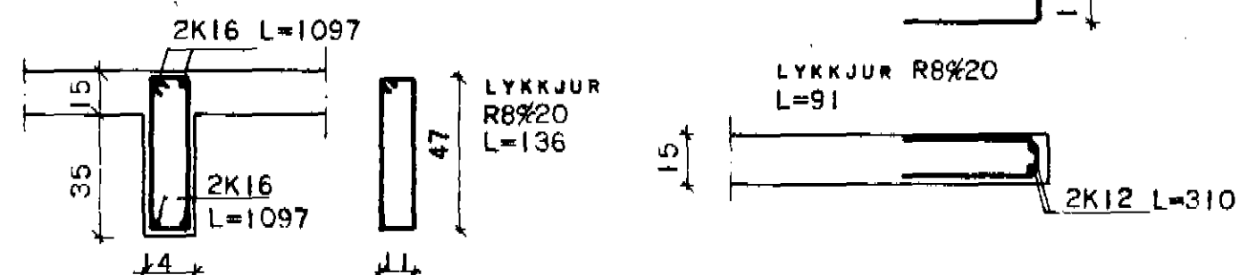
SNIB Í BITA B1 1:20
