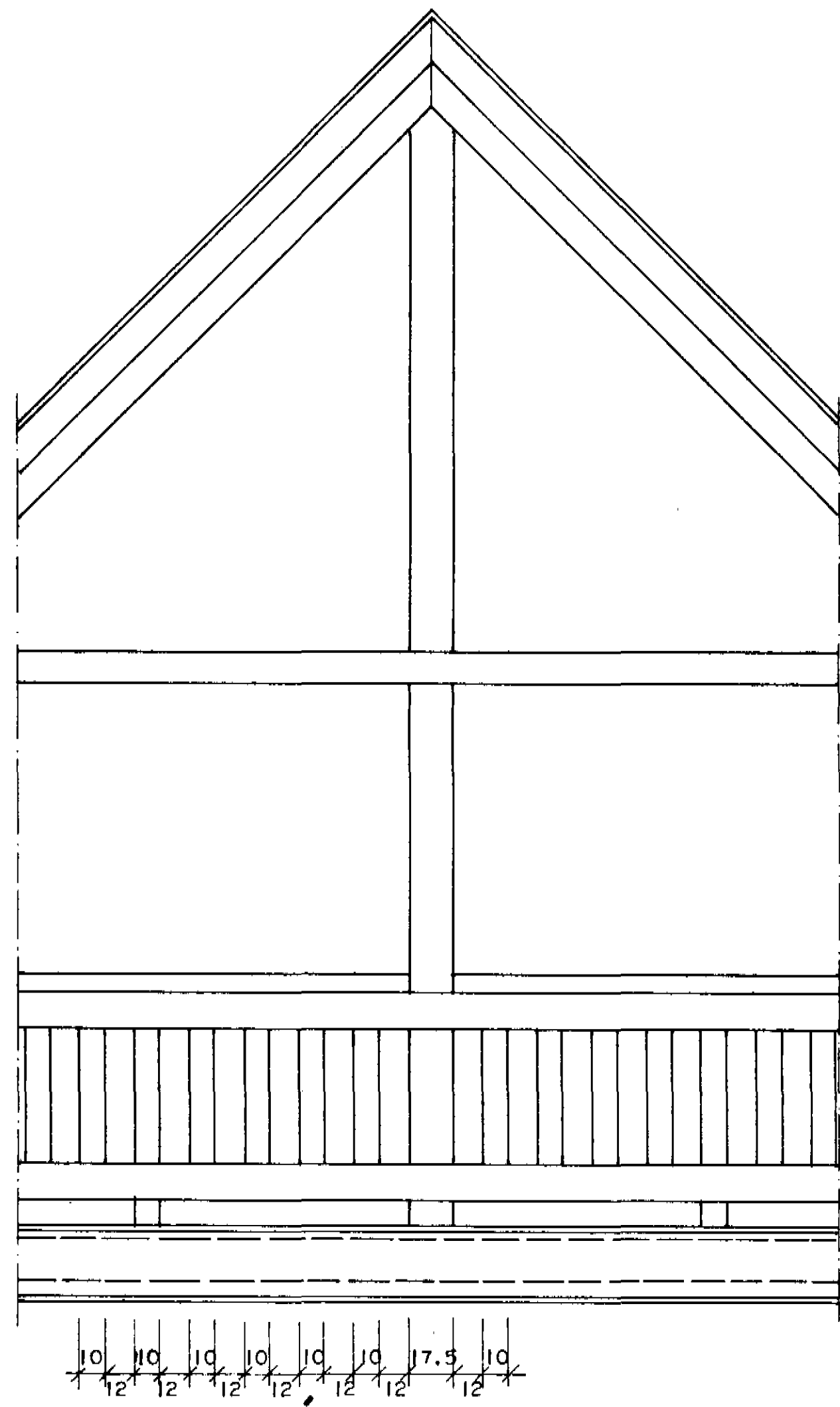
SVALAHANDRIÐ - ÚTLIT
