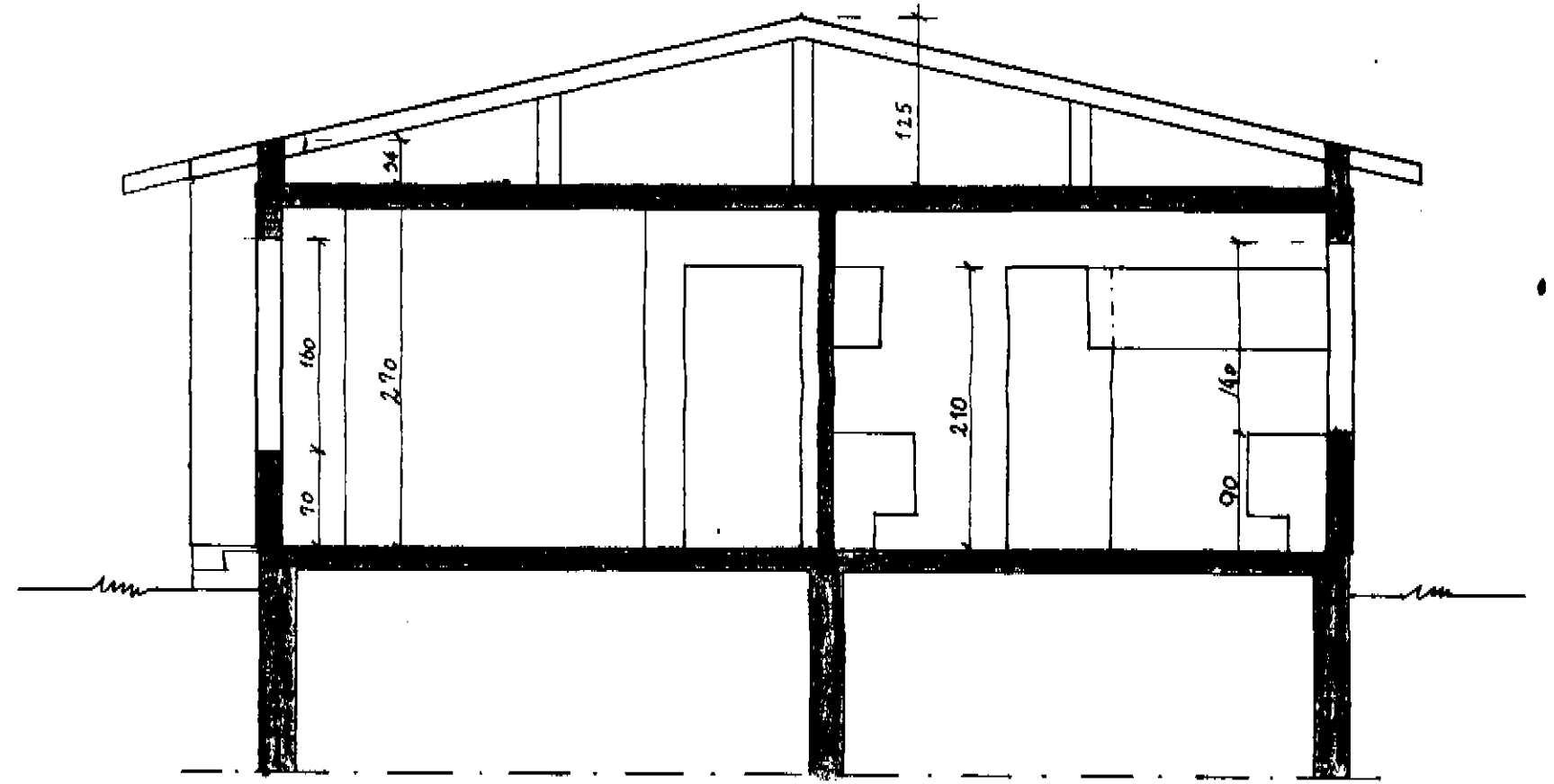
Þversnið
