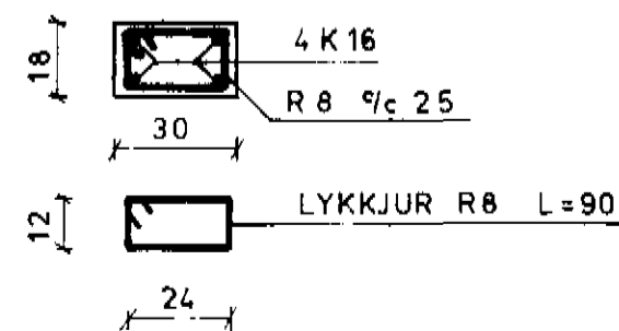
SNID Í SÚLU S-1 1:20
