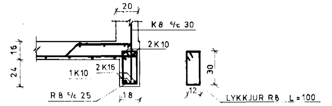
SNID A-A 1:20
