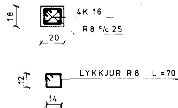
SNID Í SÚLU S-2 1:20
