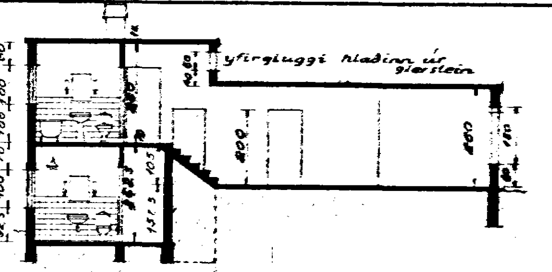
Sneiðing A-A
