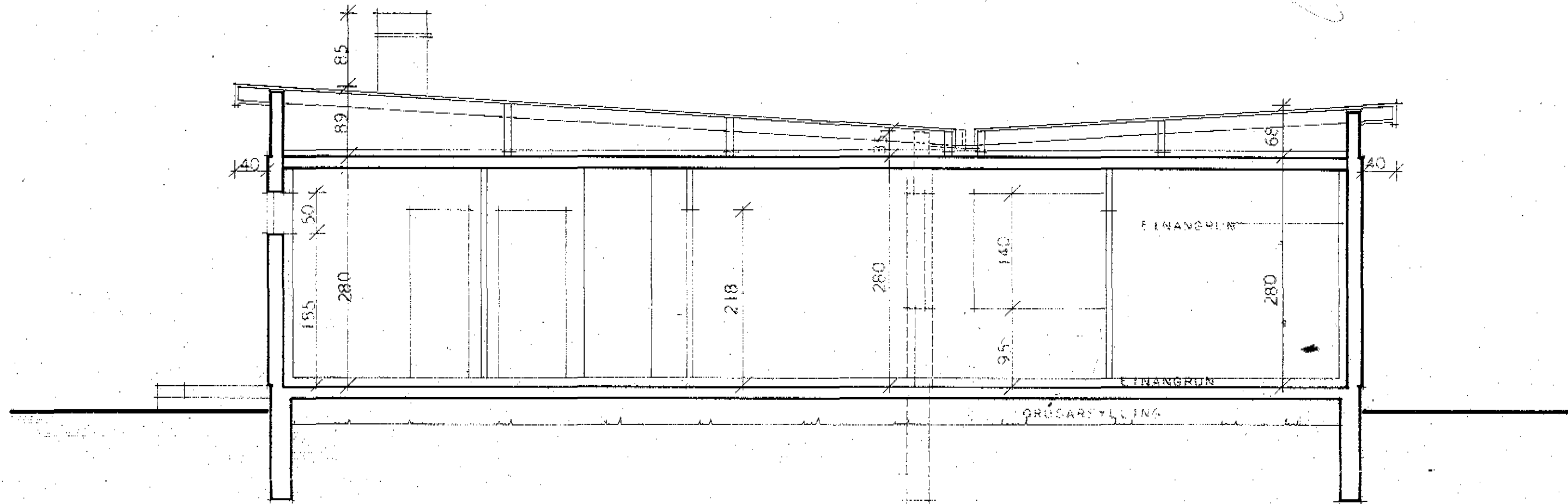
SNEIÐING A - A
