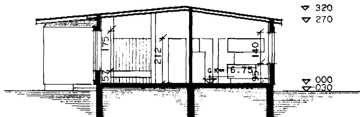
SNEIDING A-A
