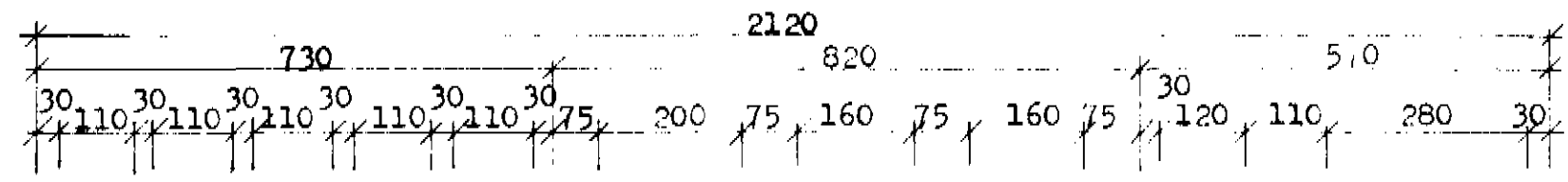
skurður A-A
