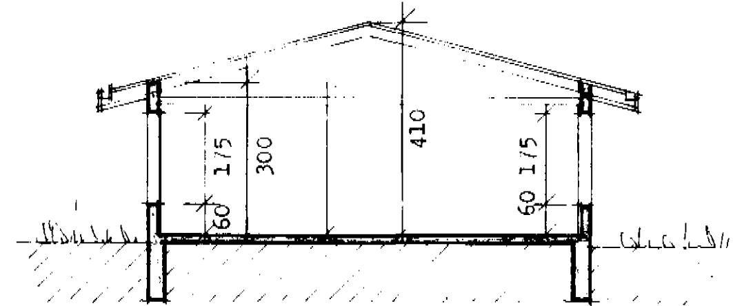
skurður B-B
