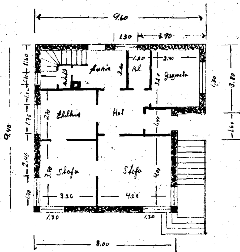
Nedri hæð
