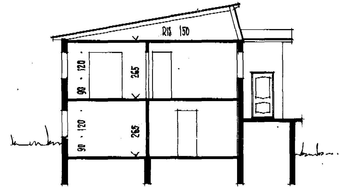
SKURÐUR 'A-A'
