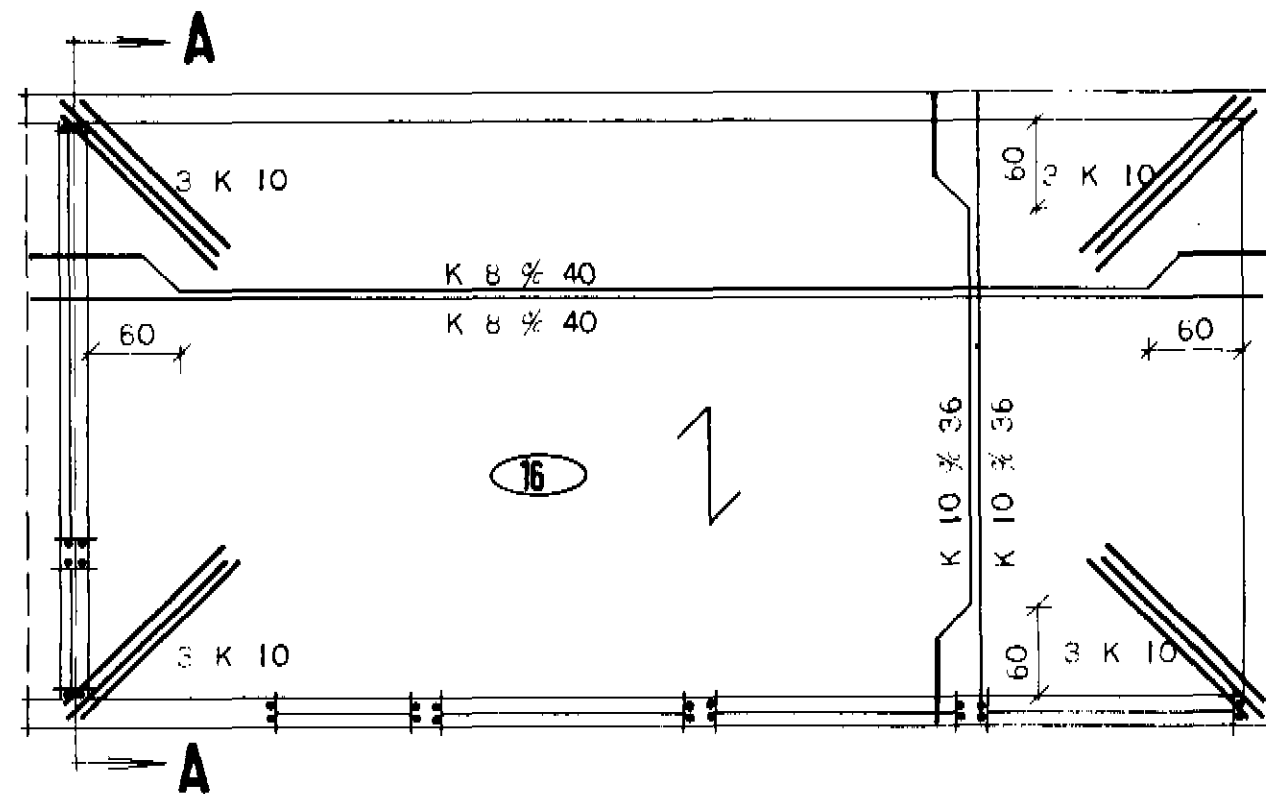
LOFTPLATA MKV. 1:50.
