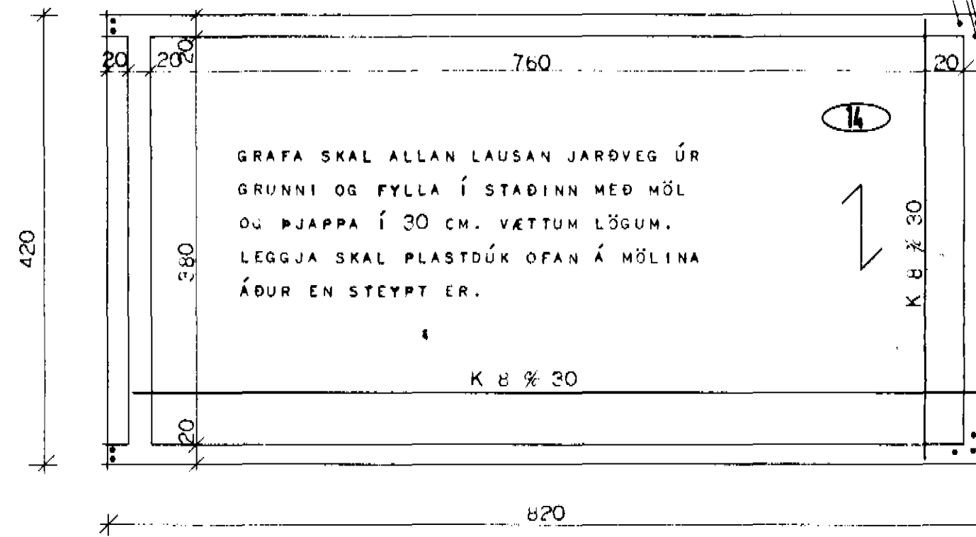
UNDIRSTÖÐUR MKV. 1:50.
