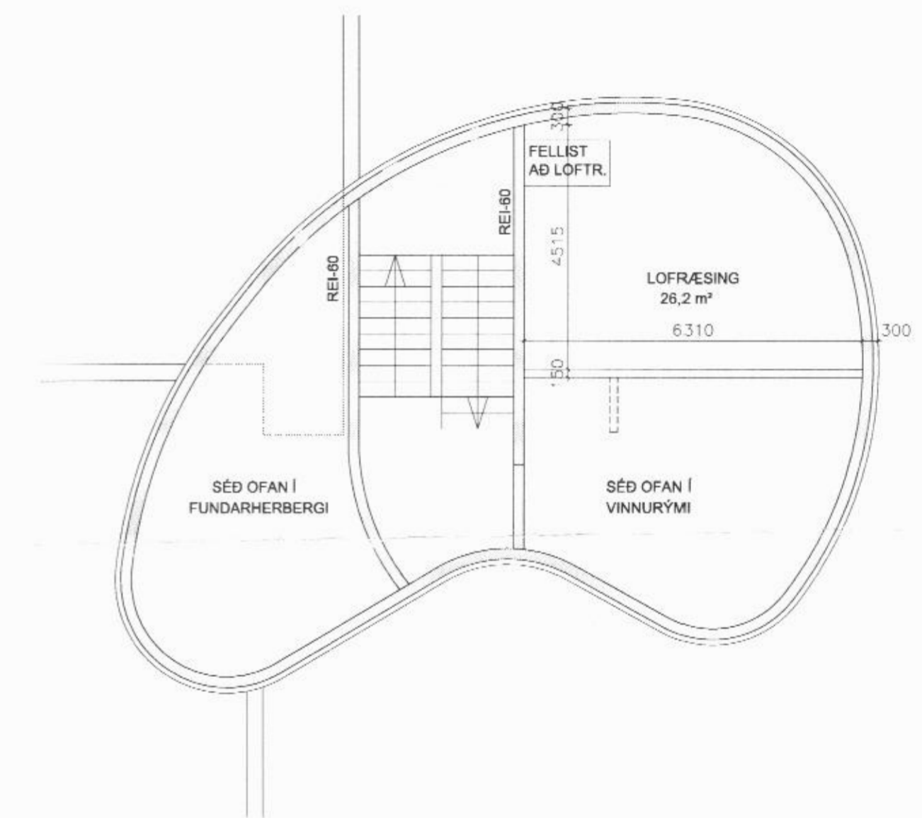
GRUNNMYND LOFRÆSIKLEFA M 1:100 @ A2
