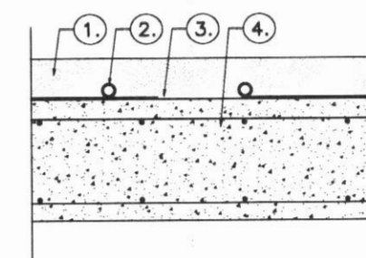
Snið í gólfgeisla. 1:10.
