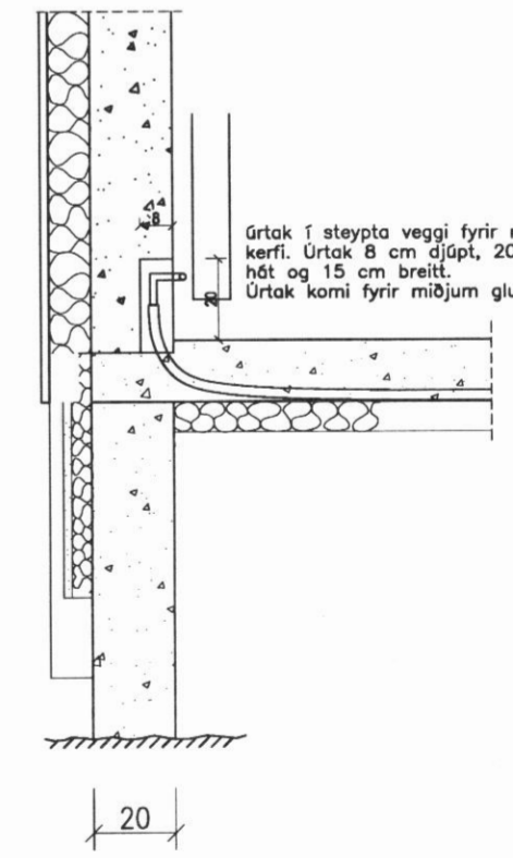
Sérmynd af úrtaki fyrir tengingu "rör í rör" - kerfis. 1:20.
