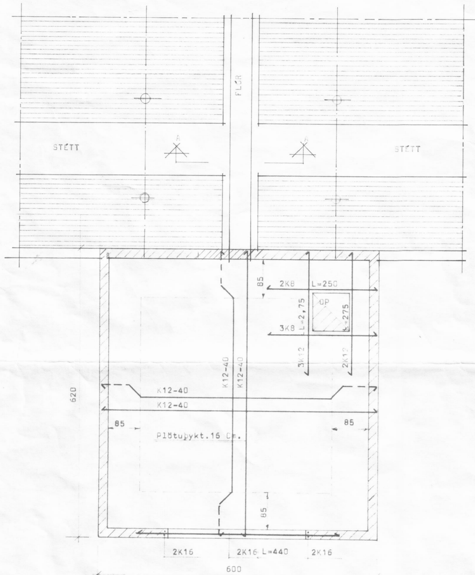
GRUNNMYND PLATA YFIR HAUGHÚS M 1:50
