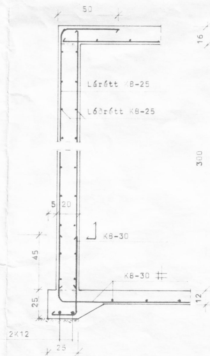
SNÍÐ Í HAUGHÚSVEGGI M 1:20
