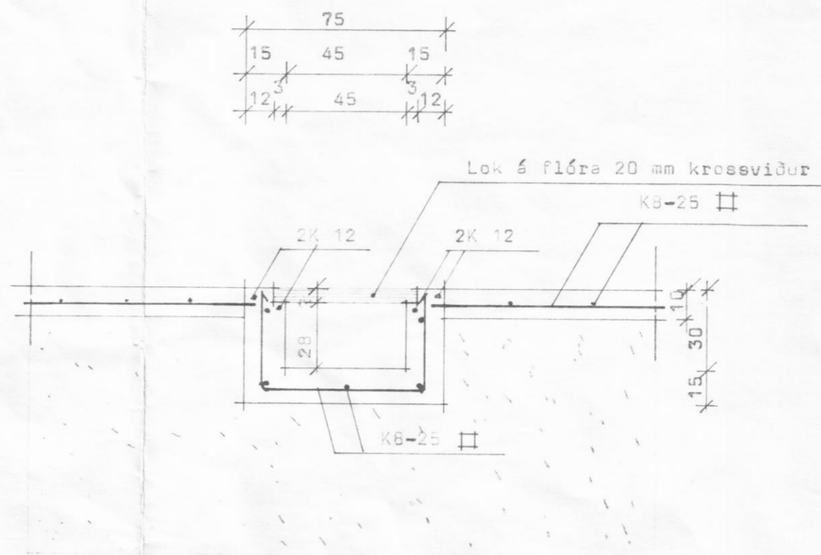
SNÍÐ Í FLÓRA OG STÉTT M 1:20
