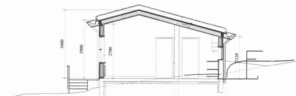
Þverskurður
