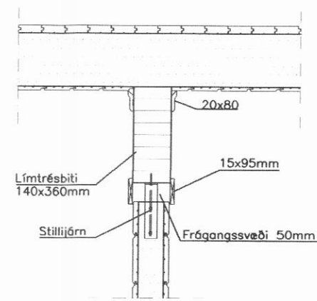
Deili 2. Mkv. 1:20
