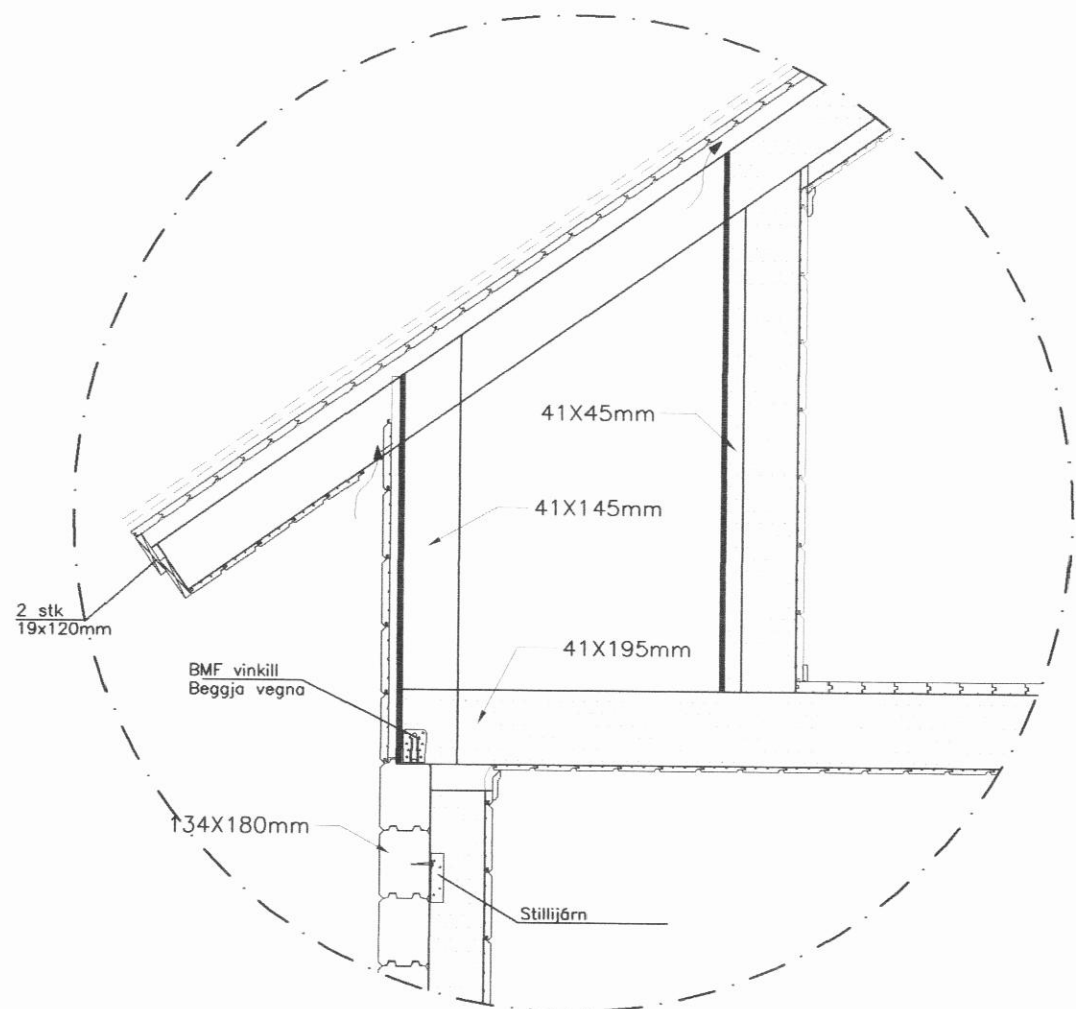
Deili 1. Mkv. 1:20
