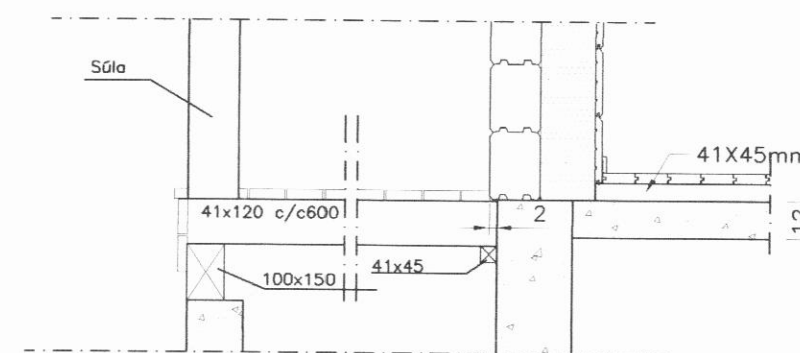
Frágangur við verönd. Mkv. 1:20
