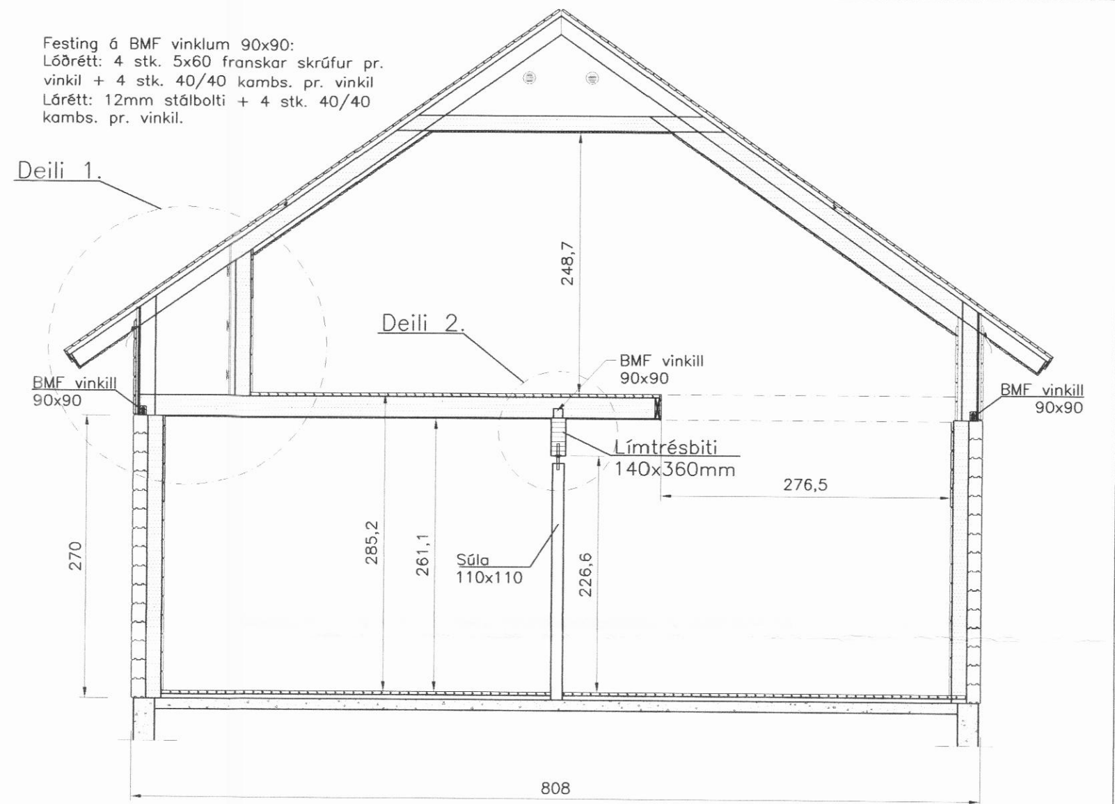
Sneiðing A-A 1:50
