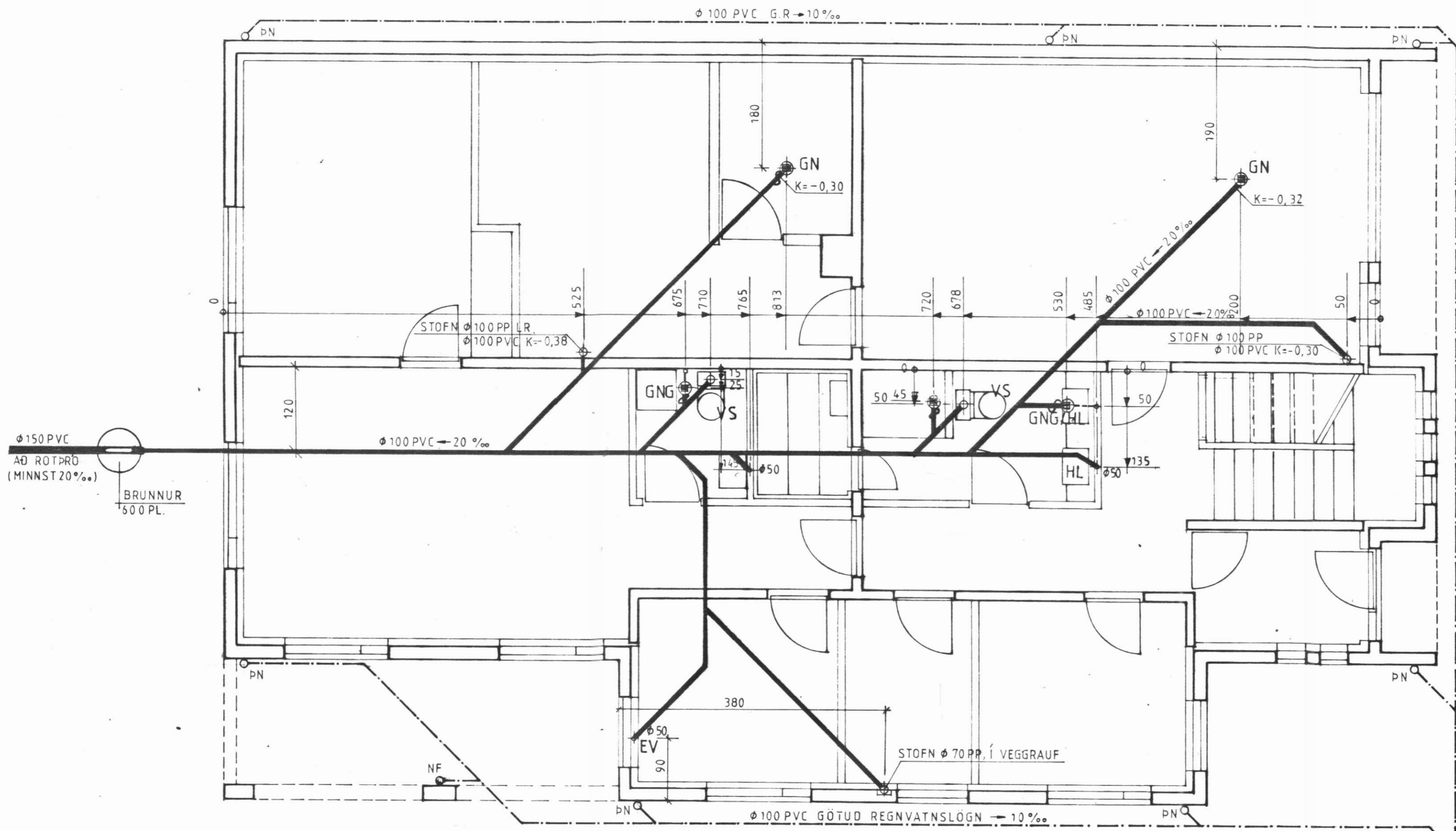
GRUNNMYND 1:50 KJALLARI
