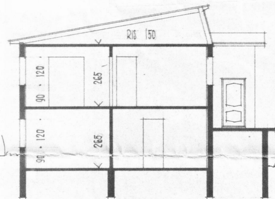
SKURÐUR "A-A"
