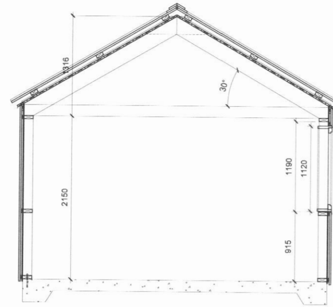
Þverskurður
