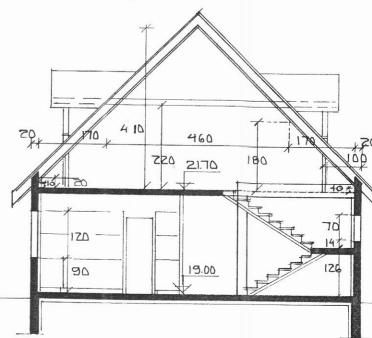
SNID A-A 1:100
