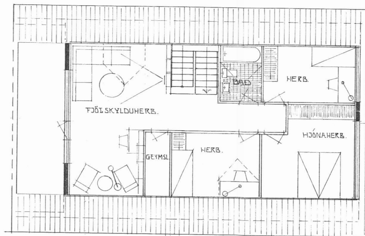
GRUNNMYND RISHEAR 1:100
