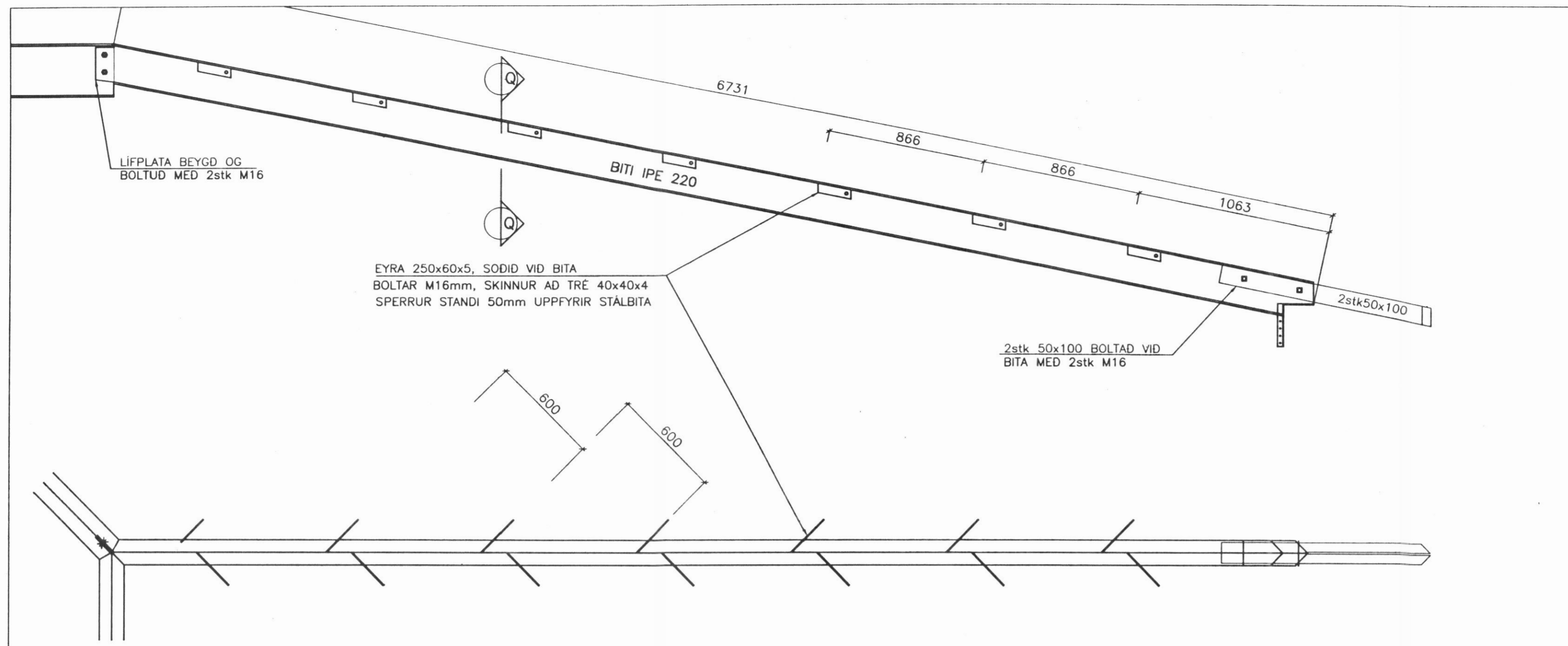
STÁLBITAR Í ÞAKI 1:20 - 2stk
