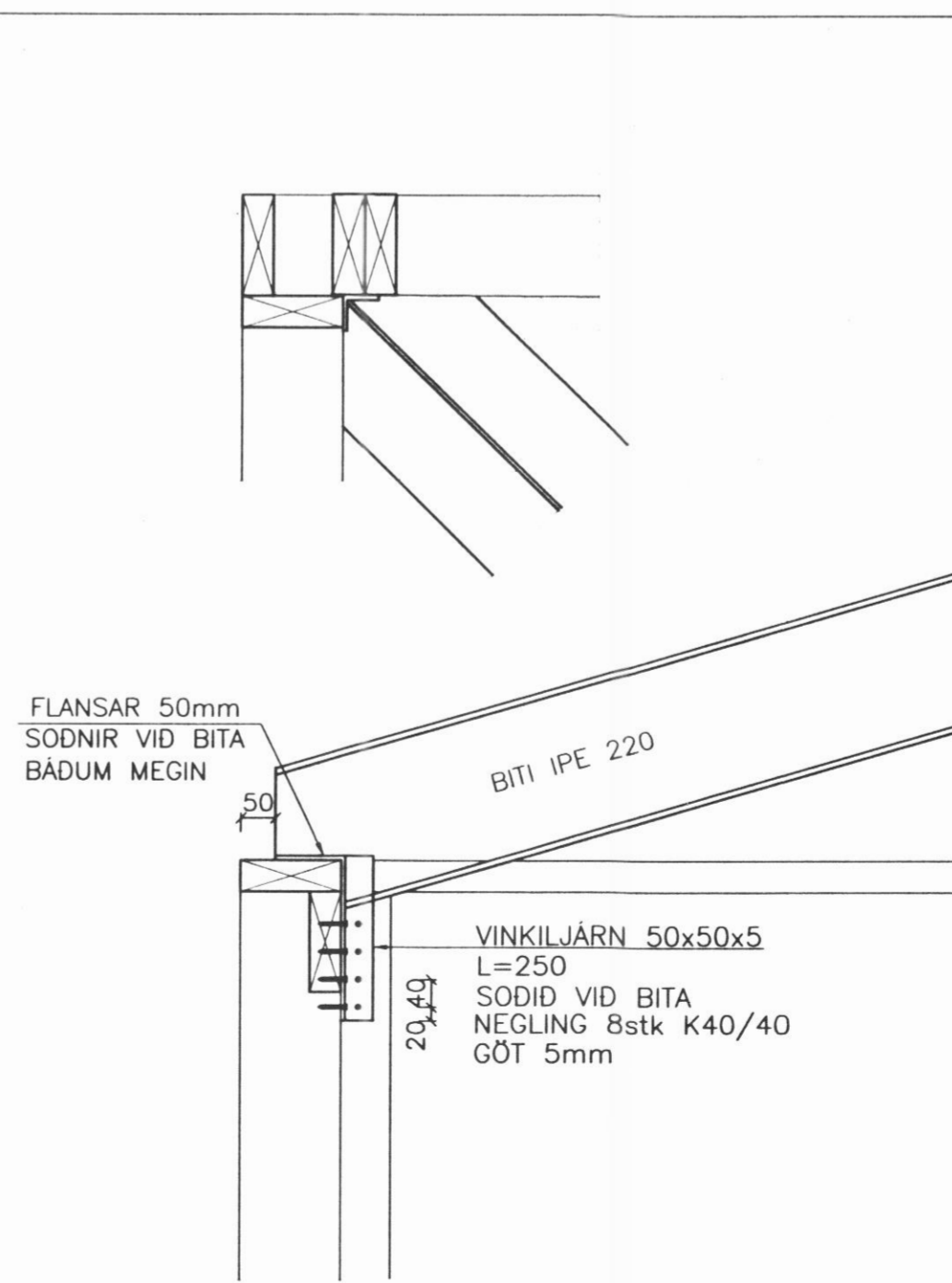
ÁSETA OG FESTING STÁLBITA Í ÚTHORNUM 1:10
