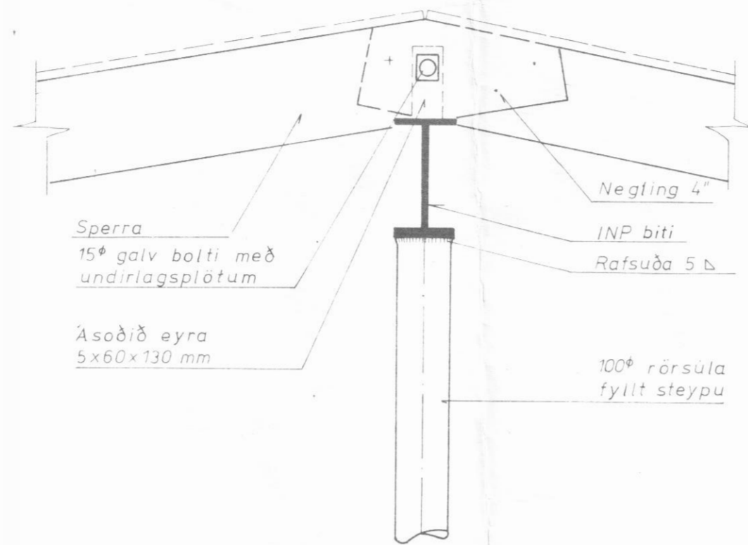
Snið B
