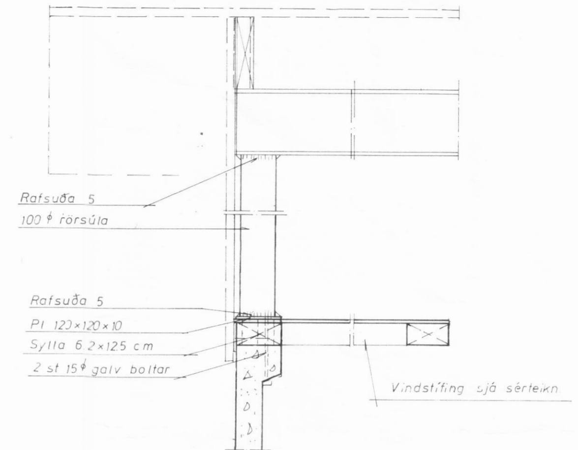
Snið C
