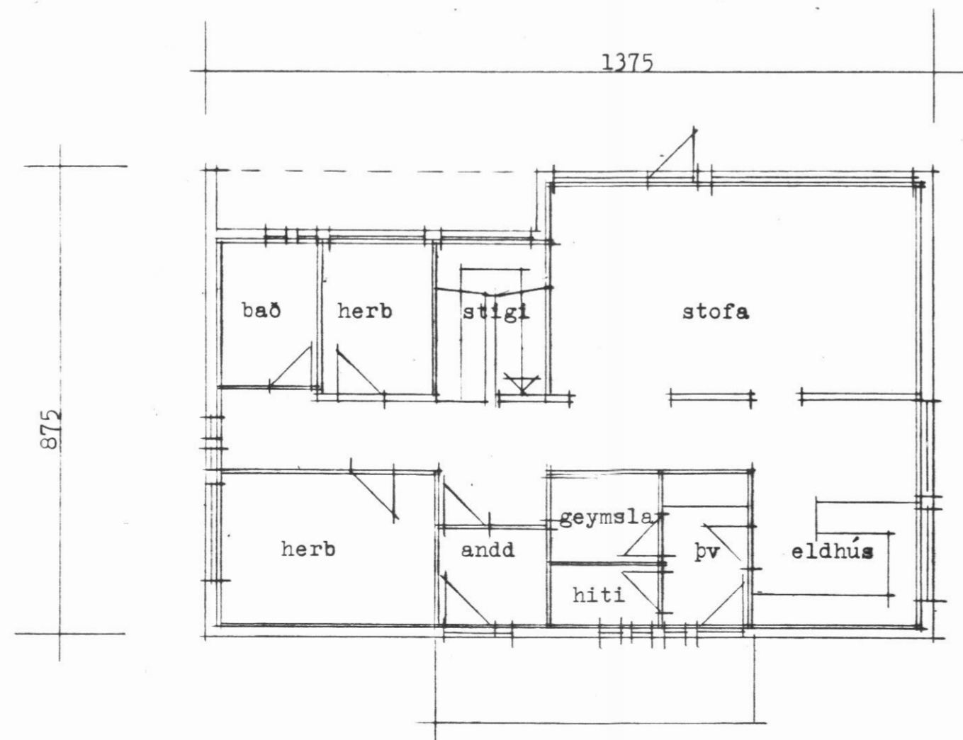
GRUNNMYND HÆÐAR mkv 1:100
