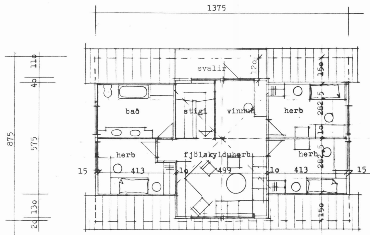
GRUNNMYND RISHÆÐAR mkv 1:100
