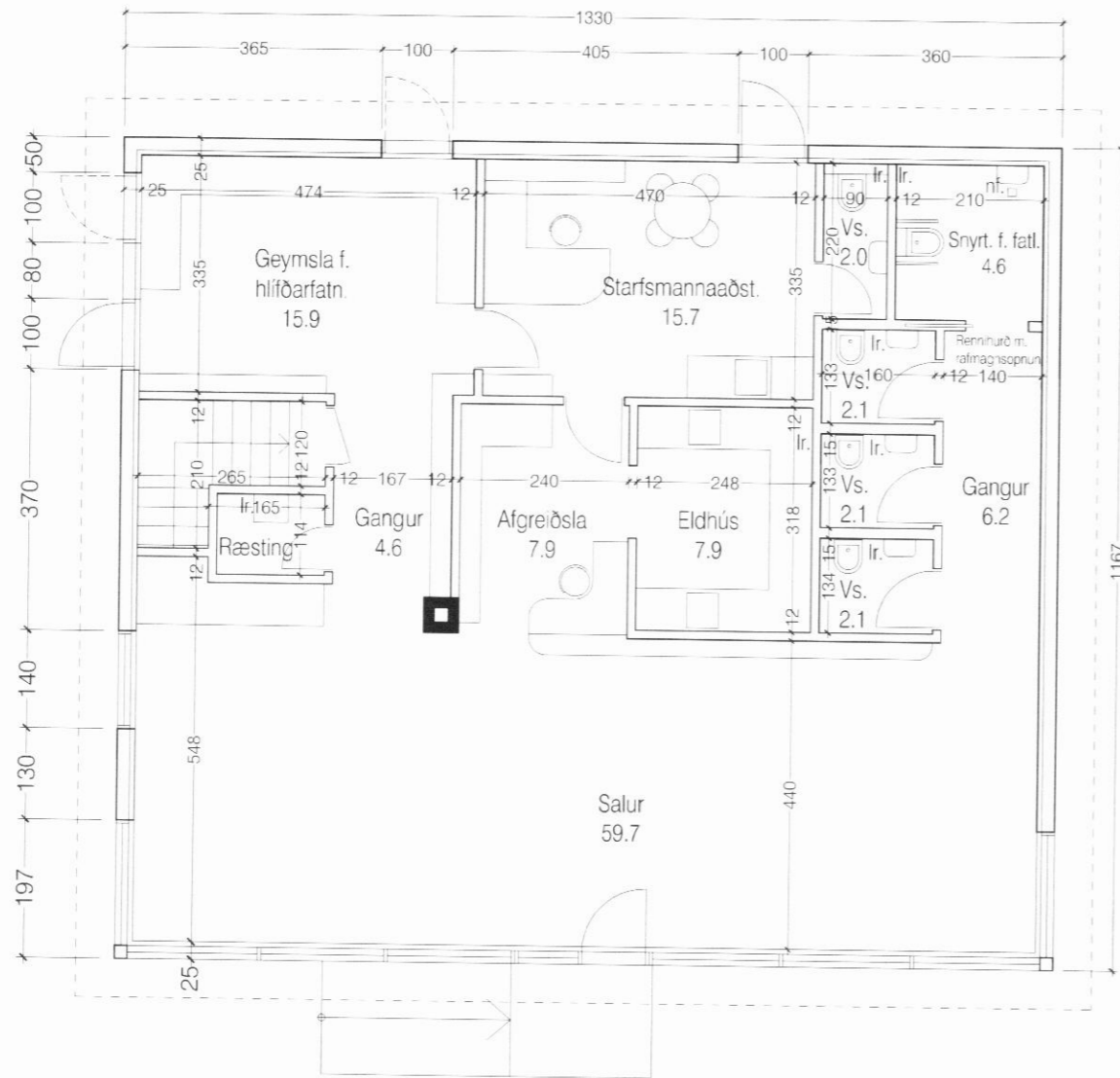
Grunnmynd jarðhæðar - mkv. 1:100
