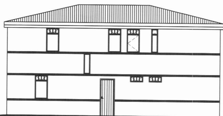
Nördurhlid 1:100
