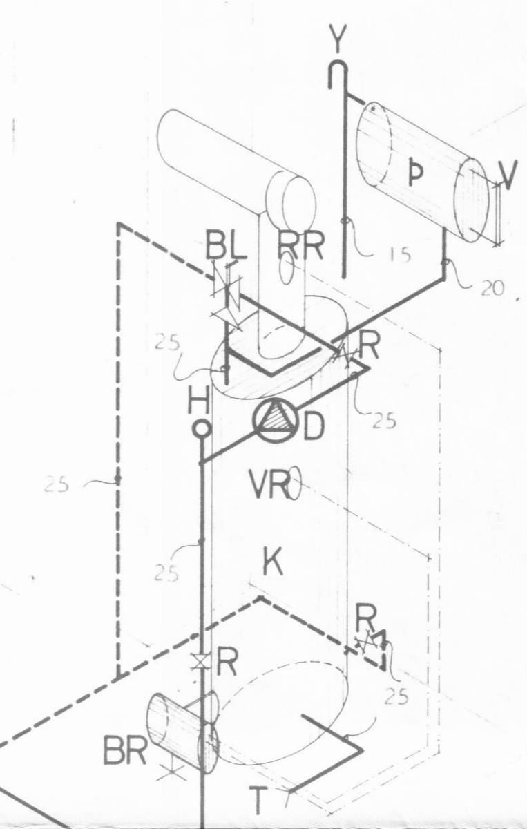
TENGIMYND AF KETILHERBERGI MKV: 1:20.
