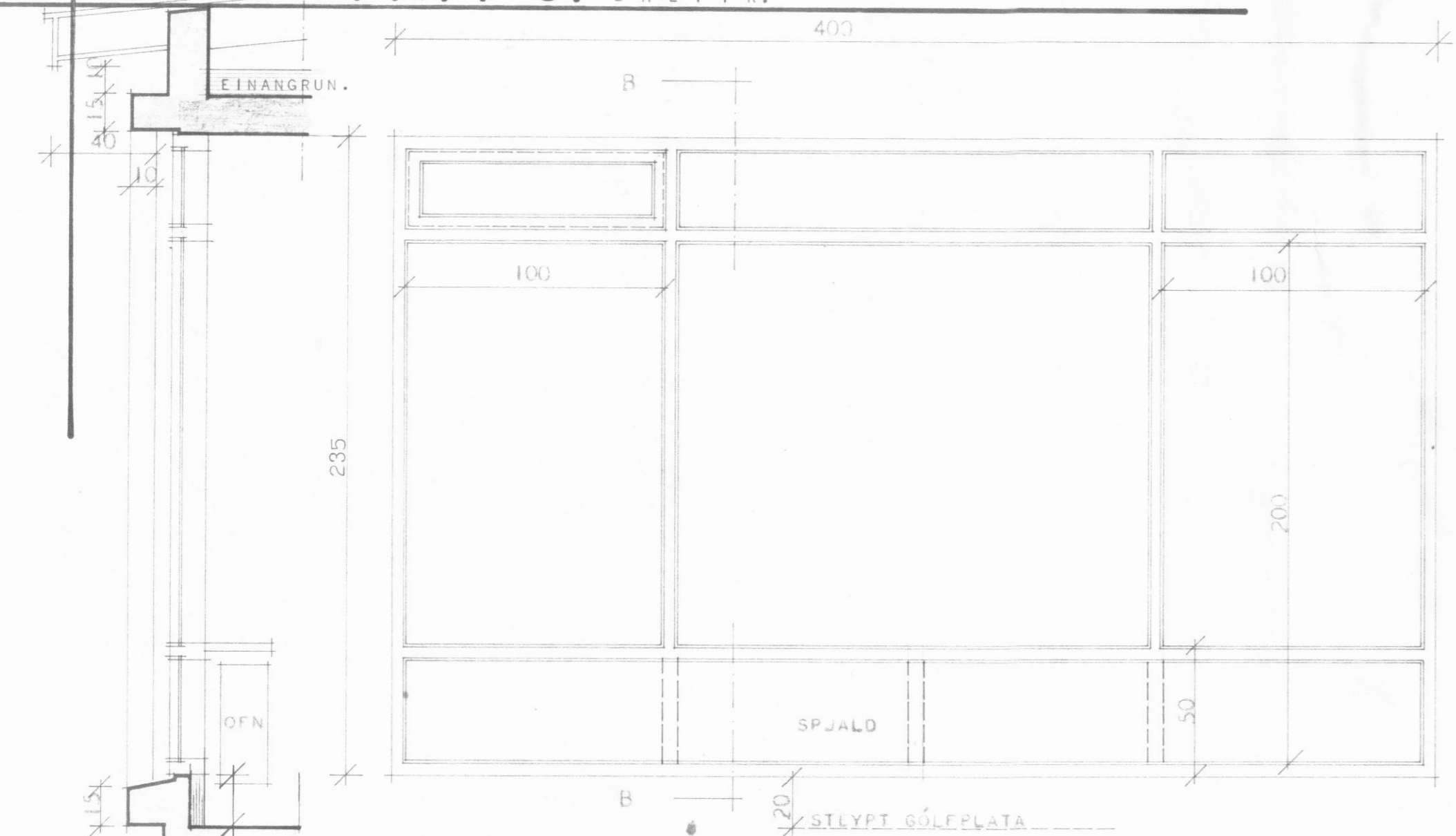
1 STK. STOFUGLUGGI.
