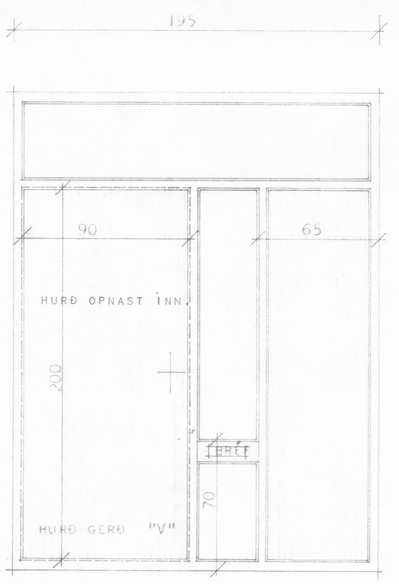
1 STK. ÚTUHURÐ. SJÁ NÁNAR BLAÐ MERKT V OG H V
