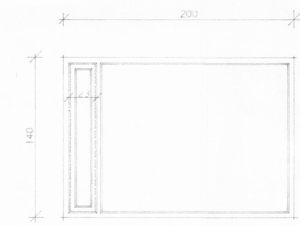
1 STK. SVÆFNHERBERGISGLUGGI.
