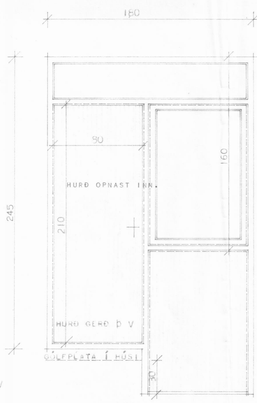
1 STK. Í ÞVOTTAHÚSI. SJÁ NÁNAR BLAÐ MERKT Þ V
