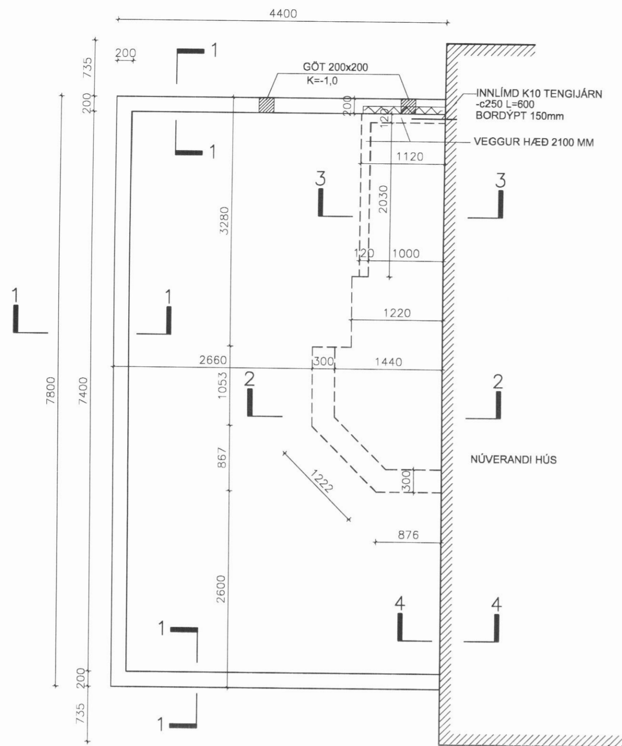
GRUNNMYND MKV. 1:50
