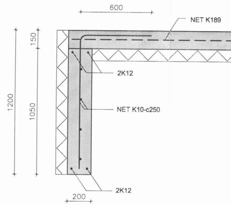
SNID 1-1 MKV. 1:20
