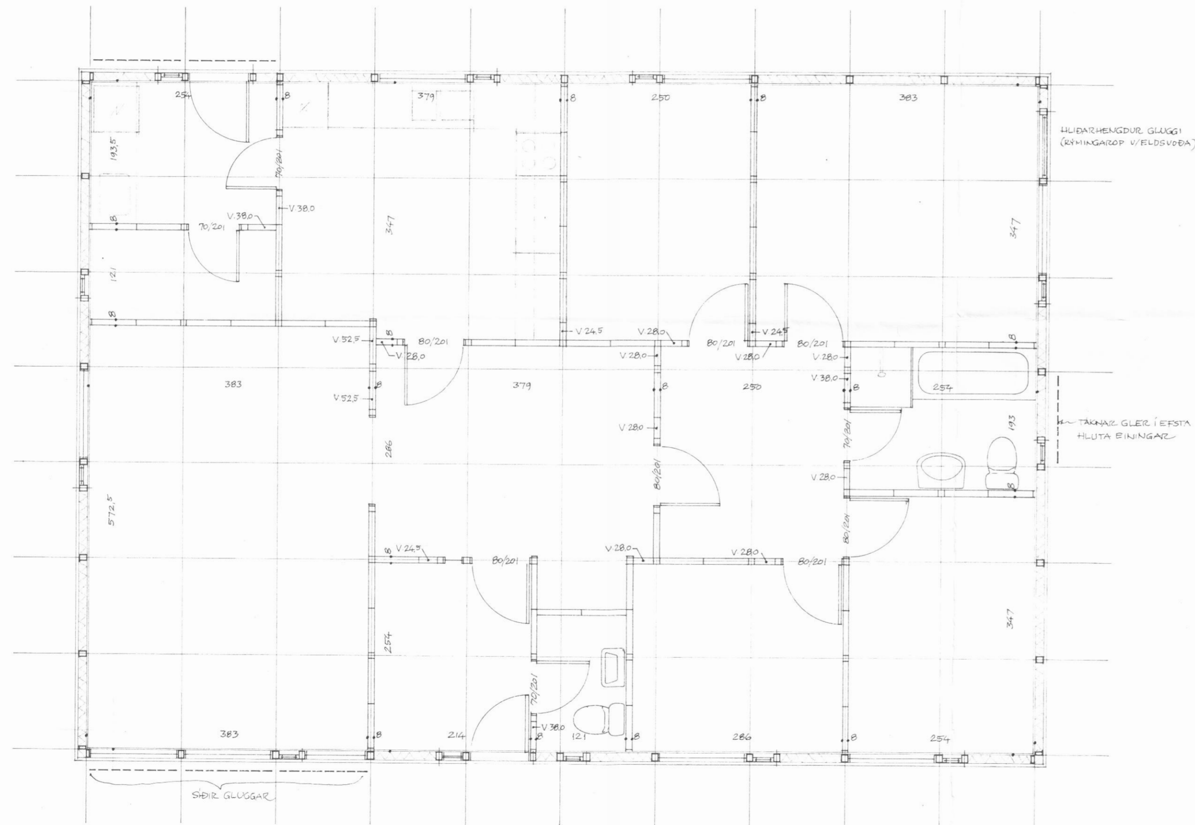
GRUNNMYND, 1:50
