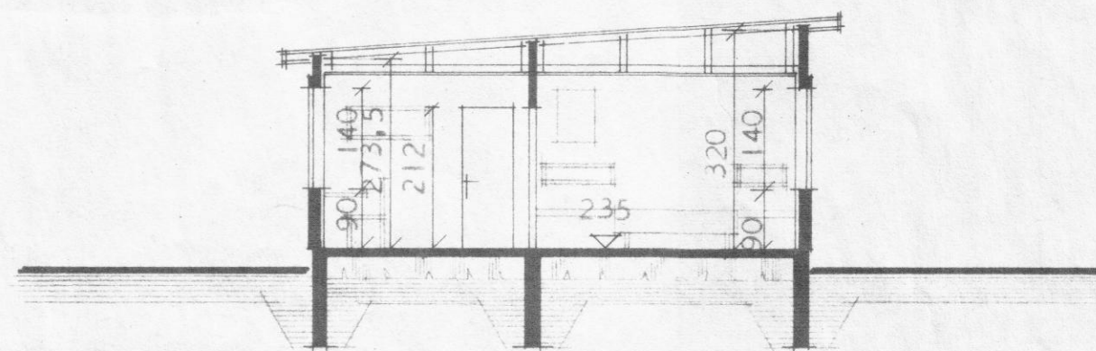
SNEIDING B---B
