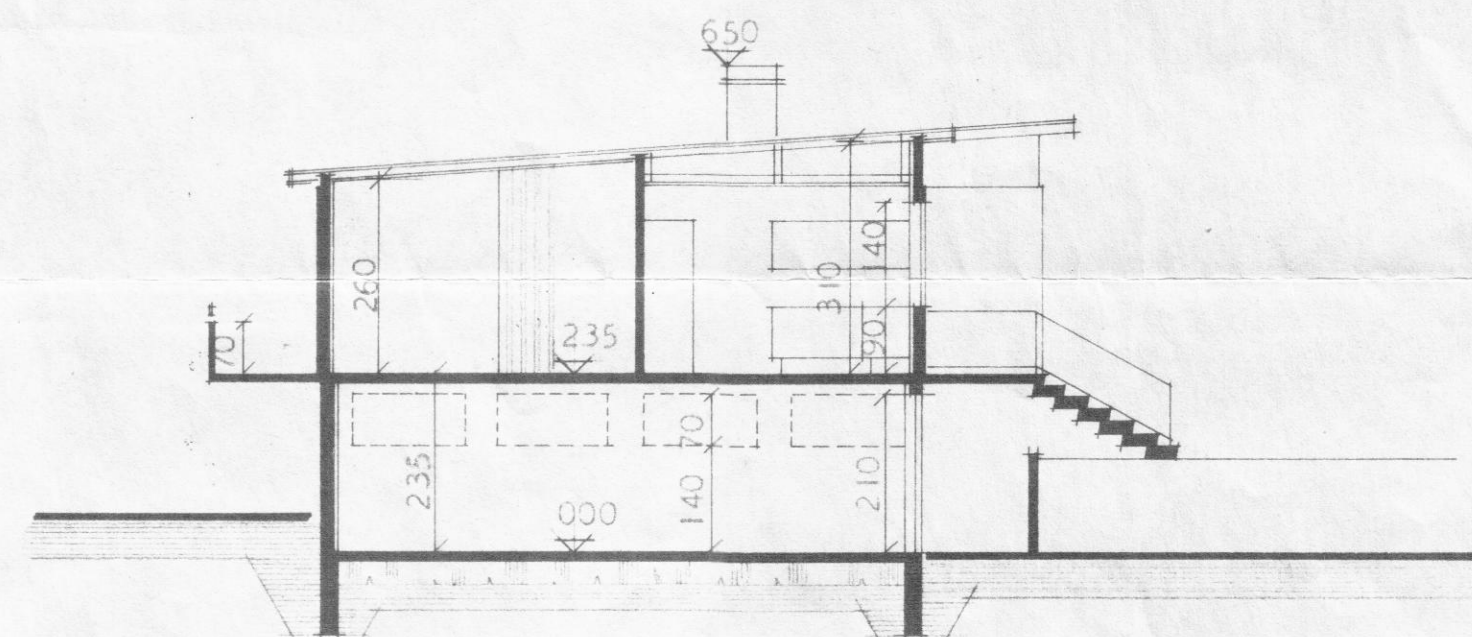
SNEIDING A---A
