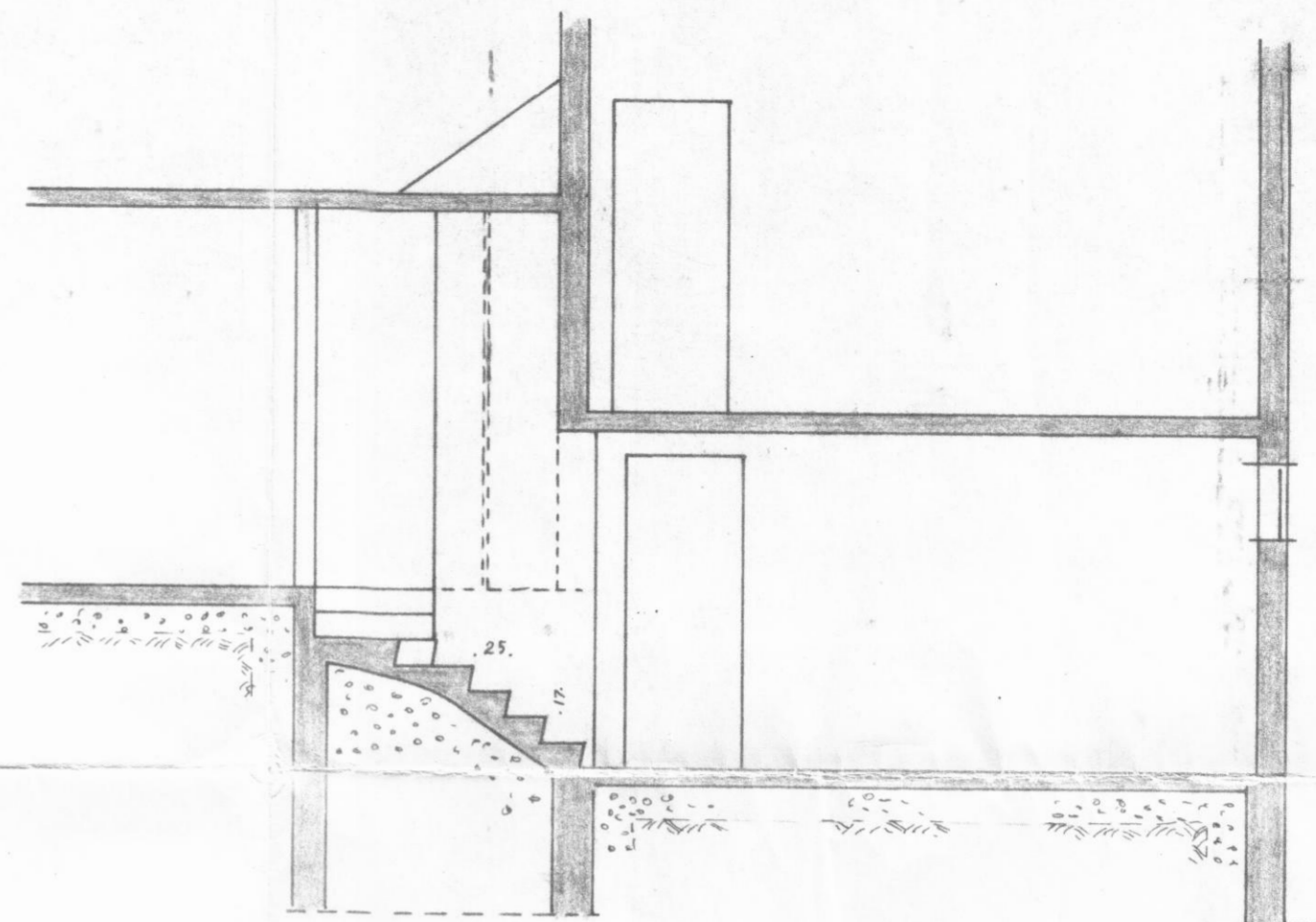
SNID B-B 1:50
