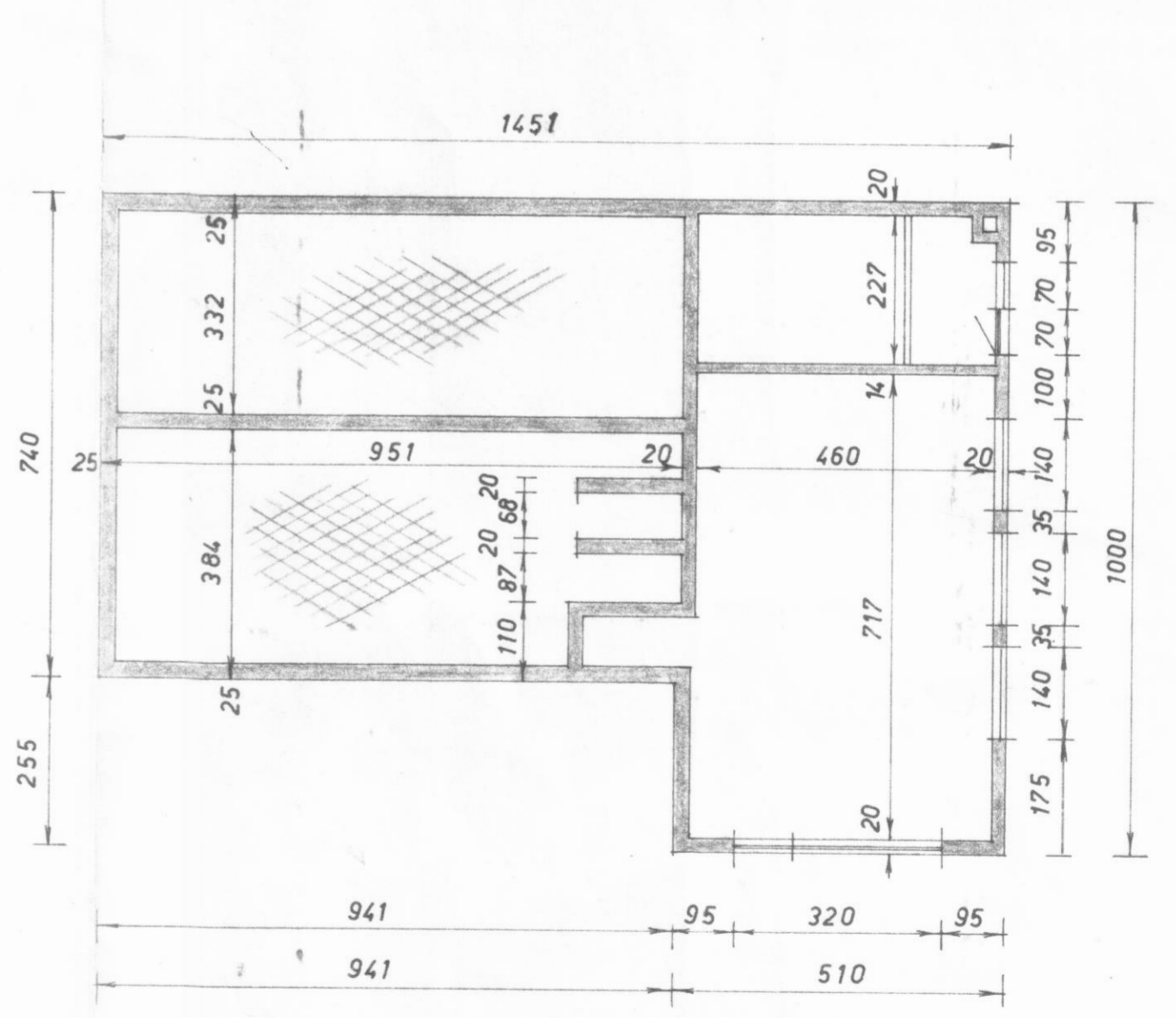
GRUNNPLAN KJALLARA 1:100
