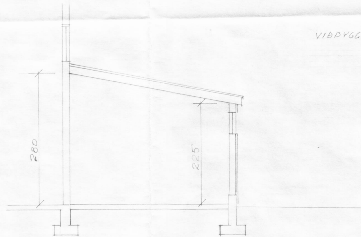
SNID M. 1:50
