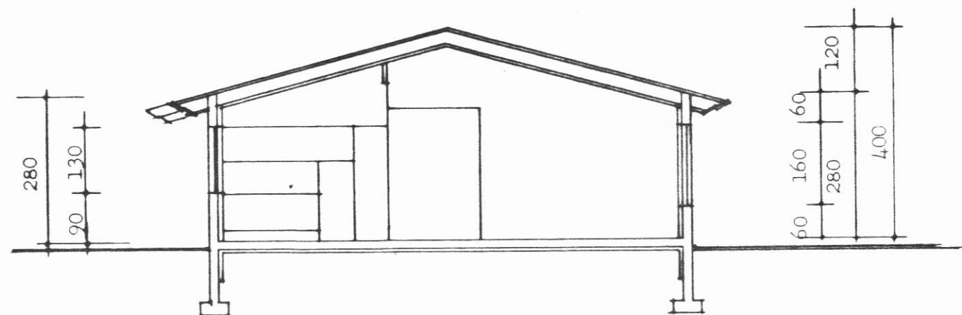
SNEIDING A - A
