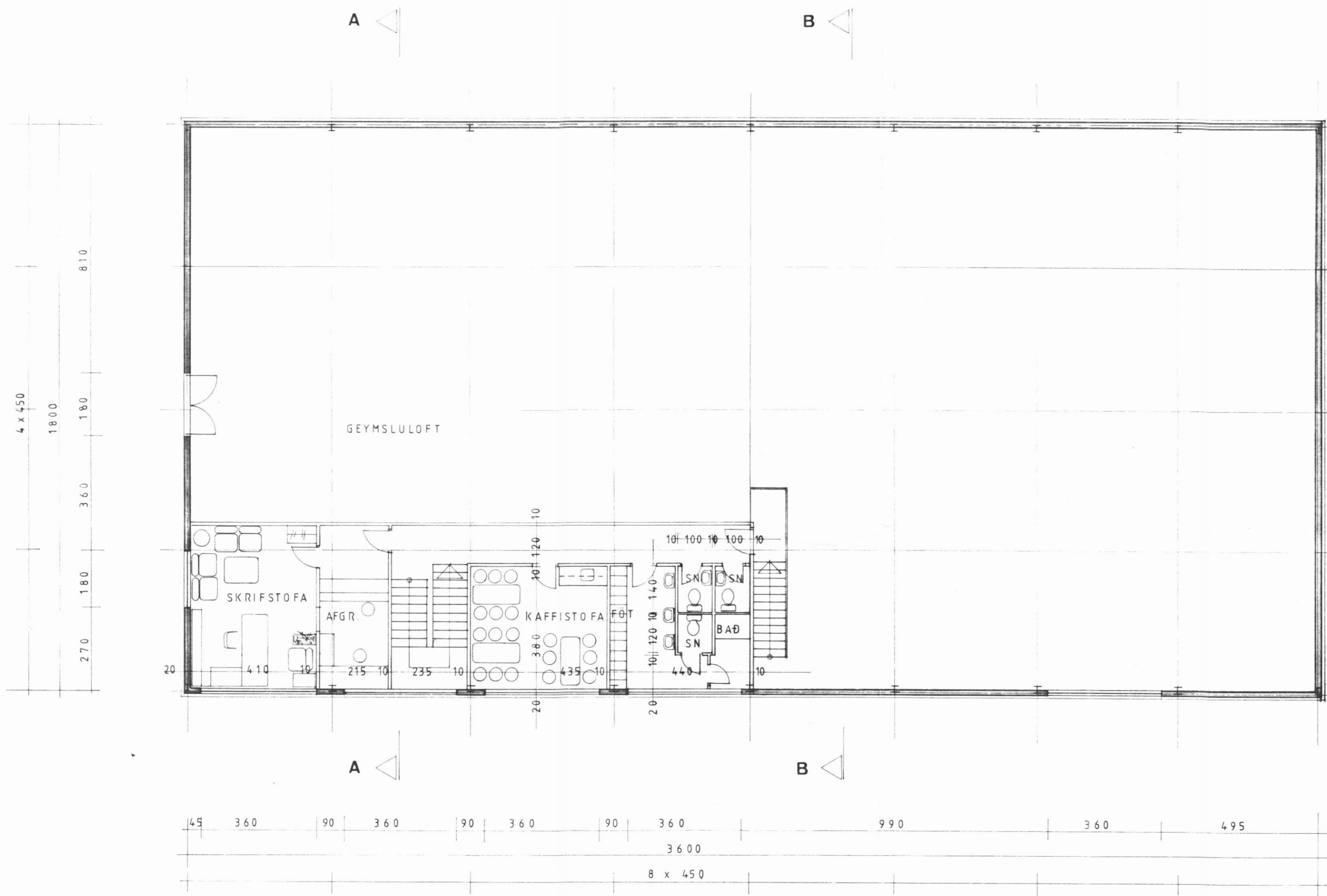
GRUNNMYND EFRI HÆÐAR 1:100
