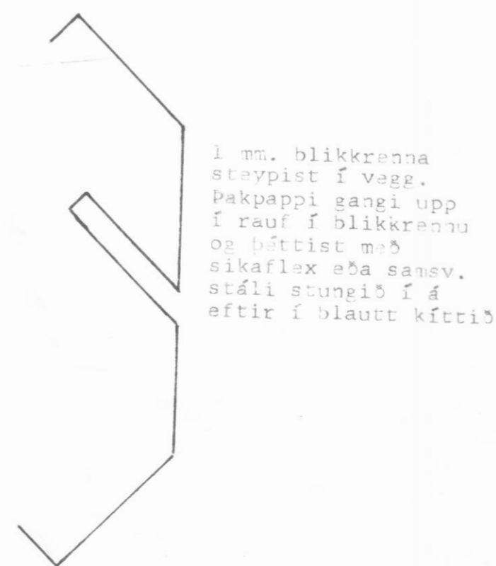
BLIKKRENNNA MK. 1:1
