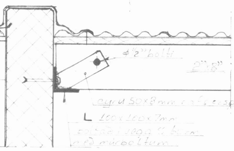
Frágangur sperra við endavegg að sunnan Snið B-B M 1:10
