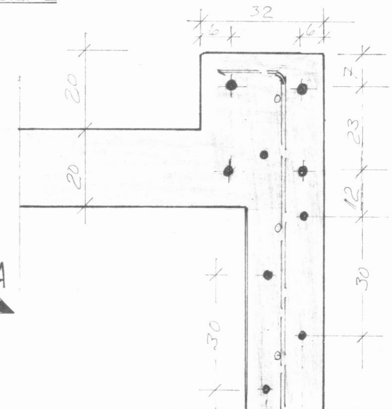
Punktur 1 staðsetning tengijärna í hornslum á norðurvegg; M 1:10
