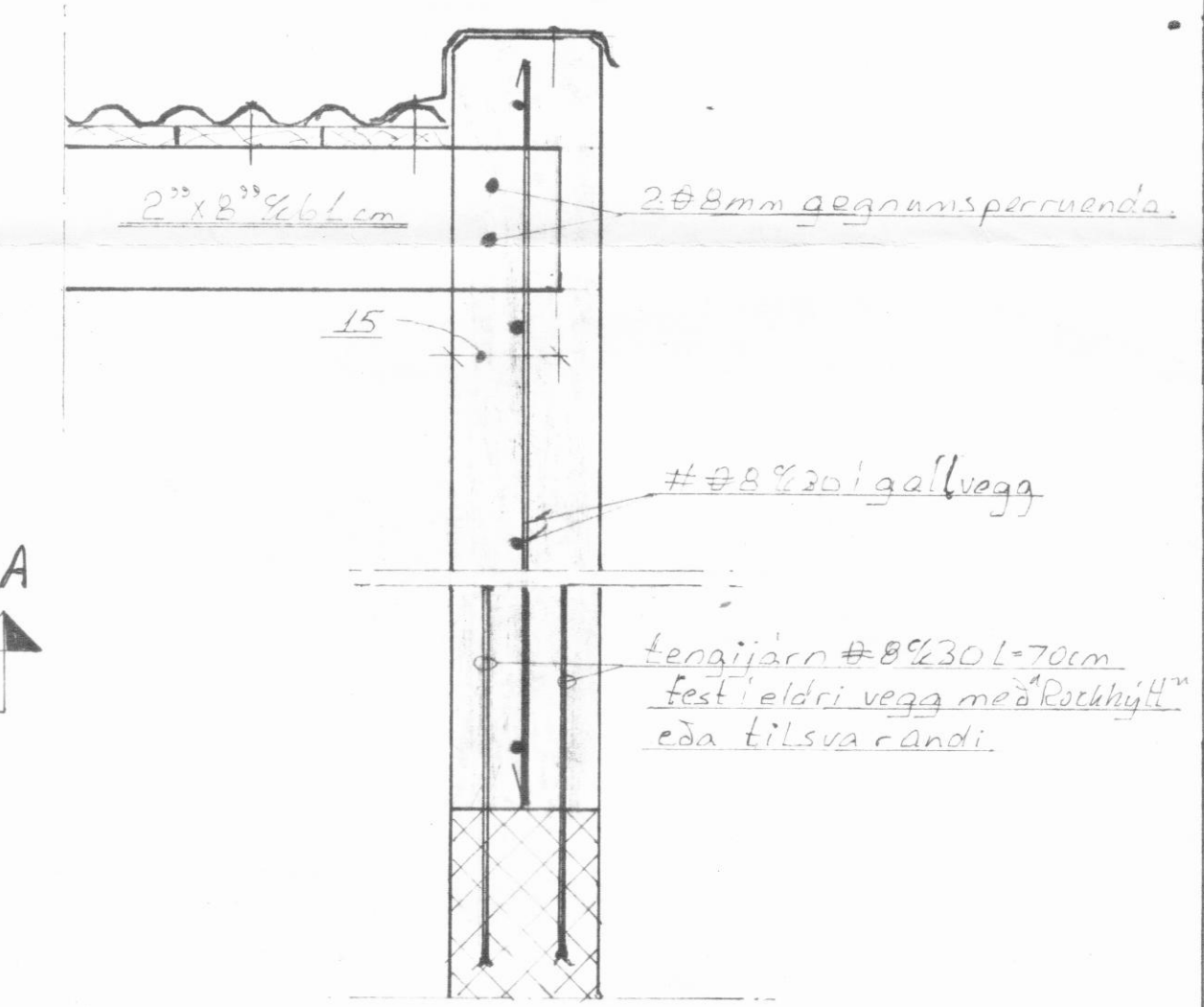
Snið A-A í endagaflað norðan M 1:10
