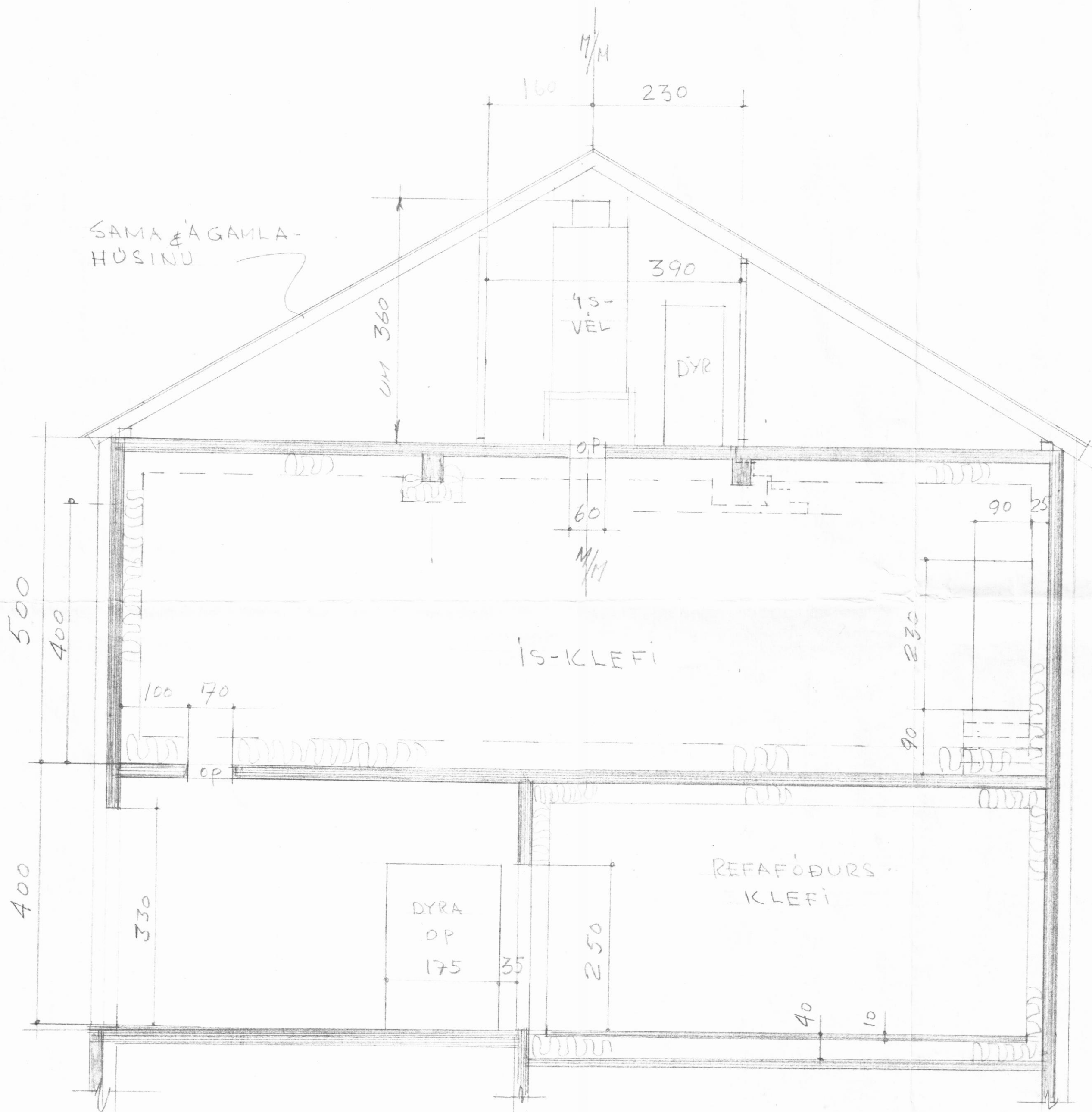
SKURÐUR "B-B" 1:50
