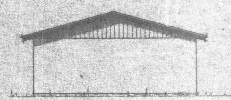
Útlit móti austri 1:100
