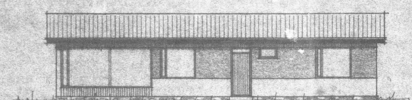
Útlit móti suðri 1:100
