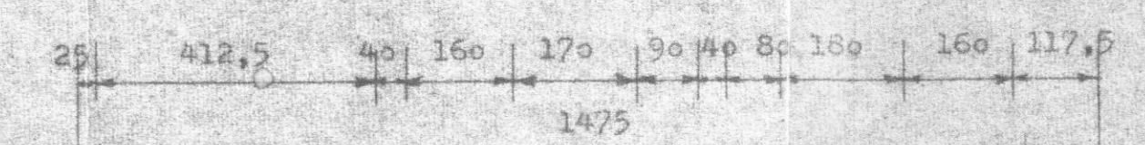
Grunnplan, 1:100 (staðsetning innveggja o.fl.)
