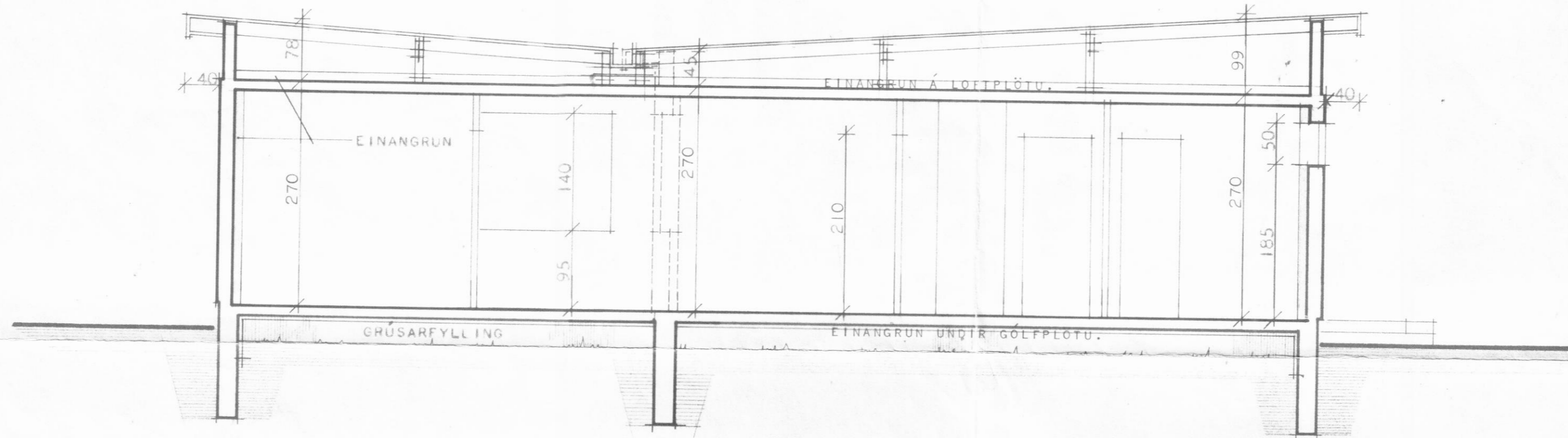
SNEIDING A-A.
