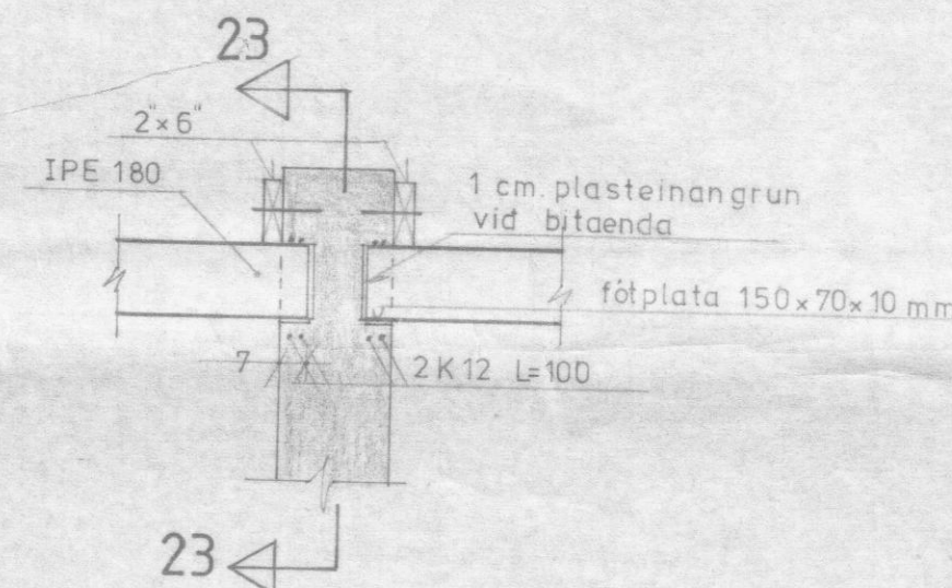
SNID 15-15 mkv. 1:20.
