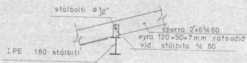
SNID 20-20, mkv. 1:20.
