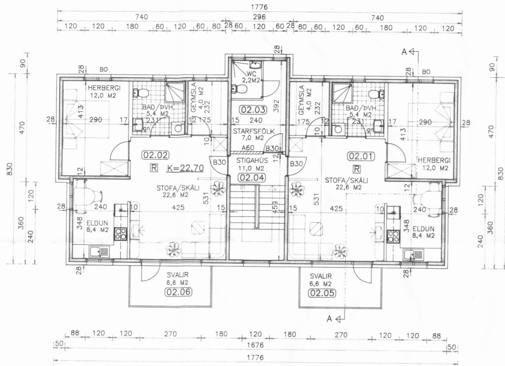
Grunnmynd efri hæðar mkv. 1:100
