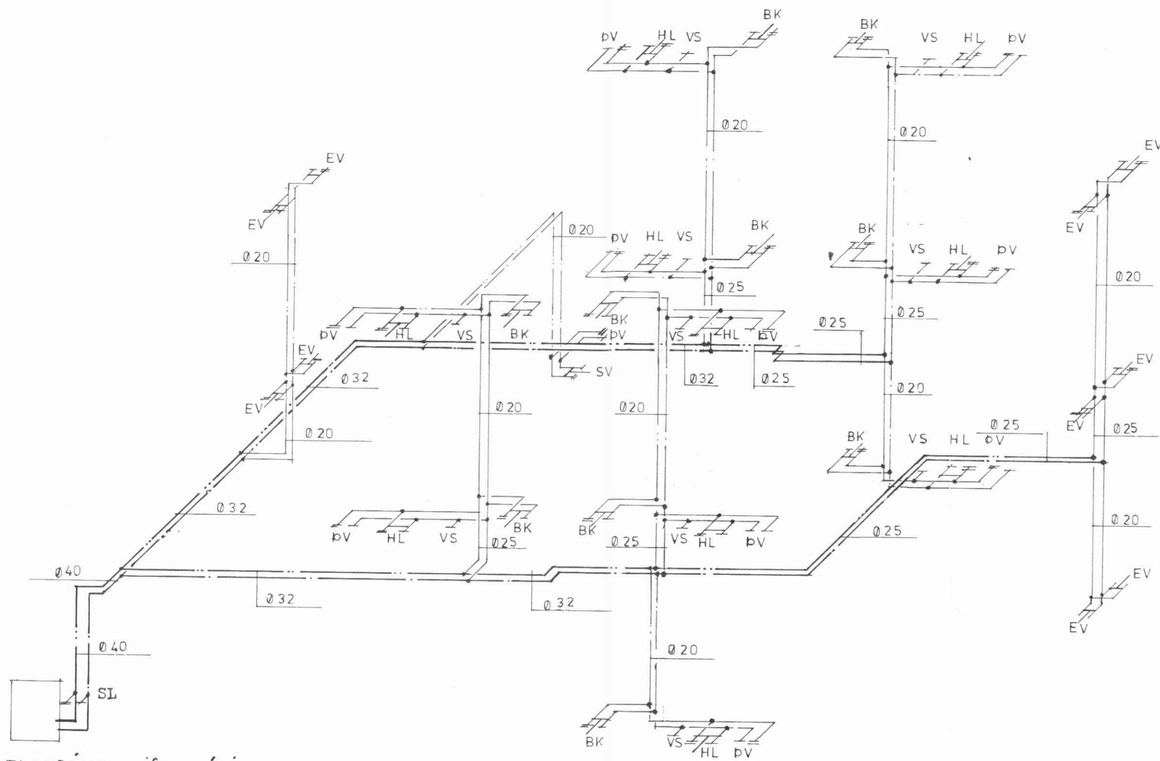
MÆLAGRIND, SJÁ SKÝRINGAMYND HITAVEITU DALVÍKUR
