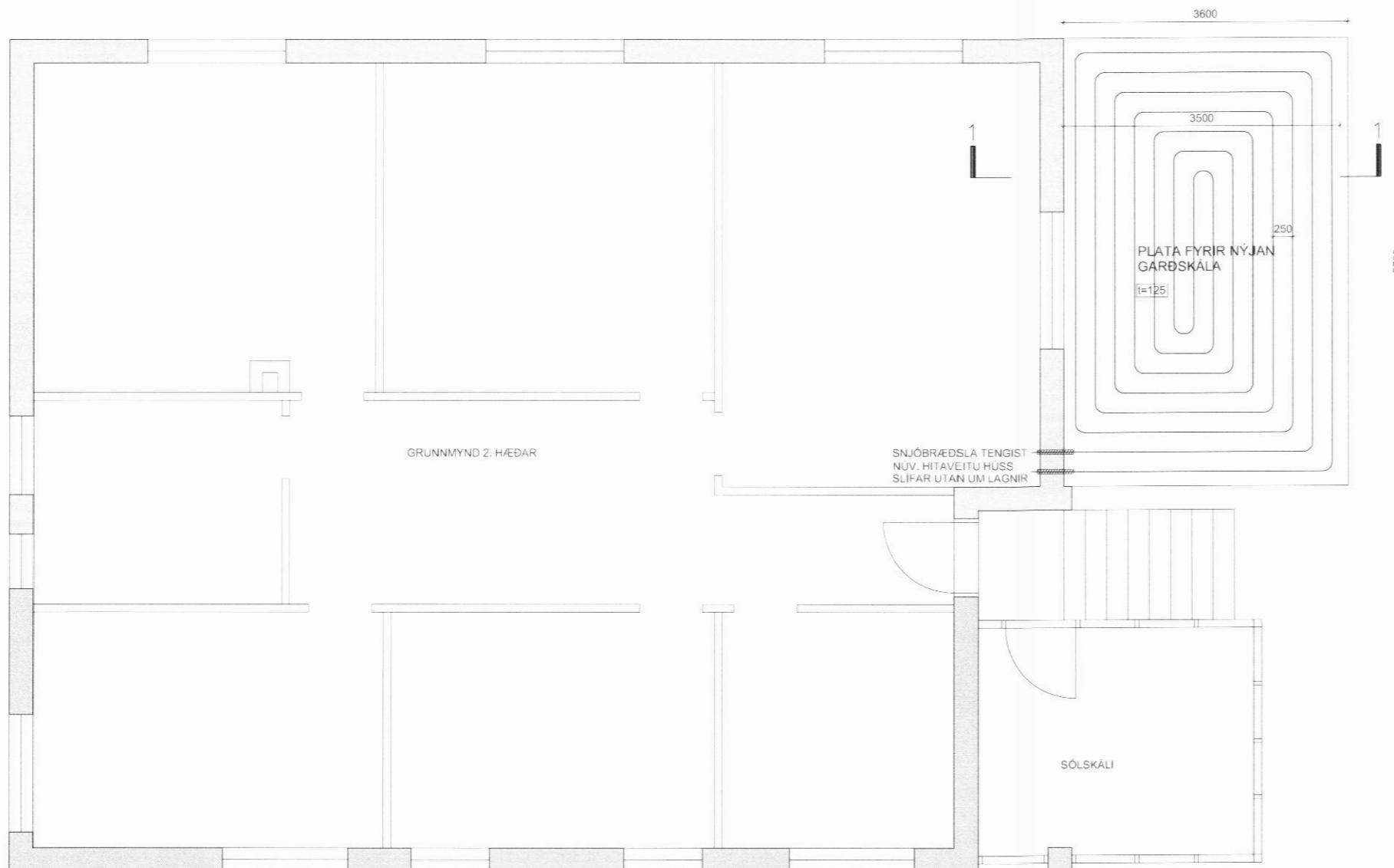
GRUNNMYND MKV. 1:50
