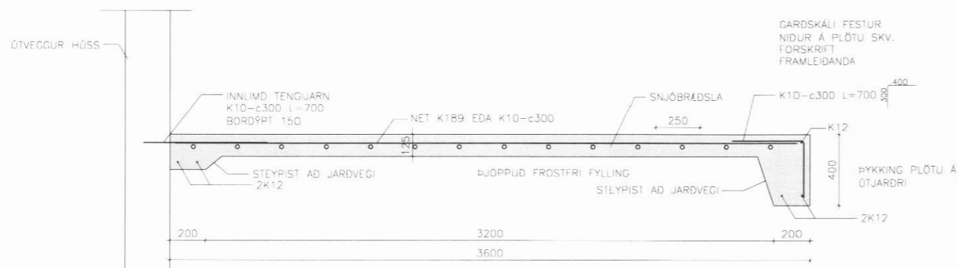
SNID 1-1 MKV. 1:20
